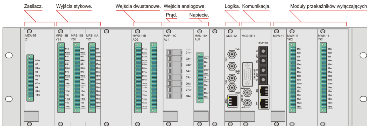
Rys. 4.6. Rozmieszczenie złączy dla przykładowego zabezpieczenia TZZ-11.
