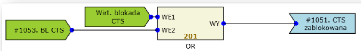
Rys. 7.31. Przykład realizacji blokady funkcji CTS.
