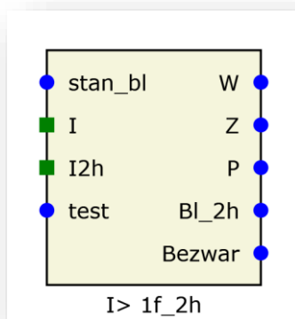
Rys. 7.14. Blok logiczny funkcji 50/51NTD.
