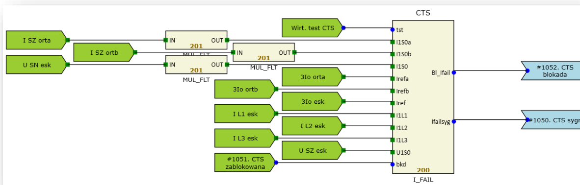
Rys. 7.30. Przykładowa konfiguracja funkcji CTS.
