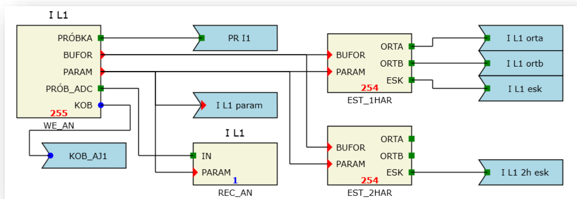
Rys. 5.18. Przykładowa konfiguracja wejścia prądowego.
