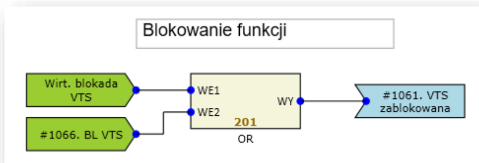
Rys. 7.27. Przykład realizacji blokady funkcji VTS.
