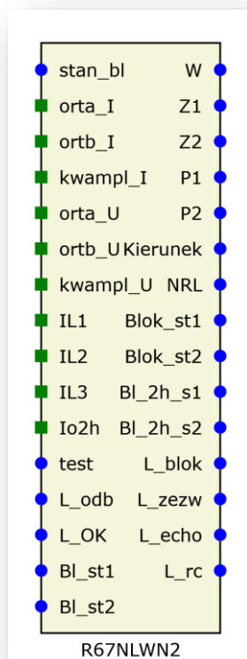
Rys. 7.6. Blok logiczny R67N_LWN2 funkcji ziemnozwarciowej (67N).
