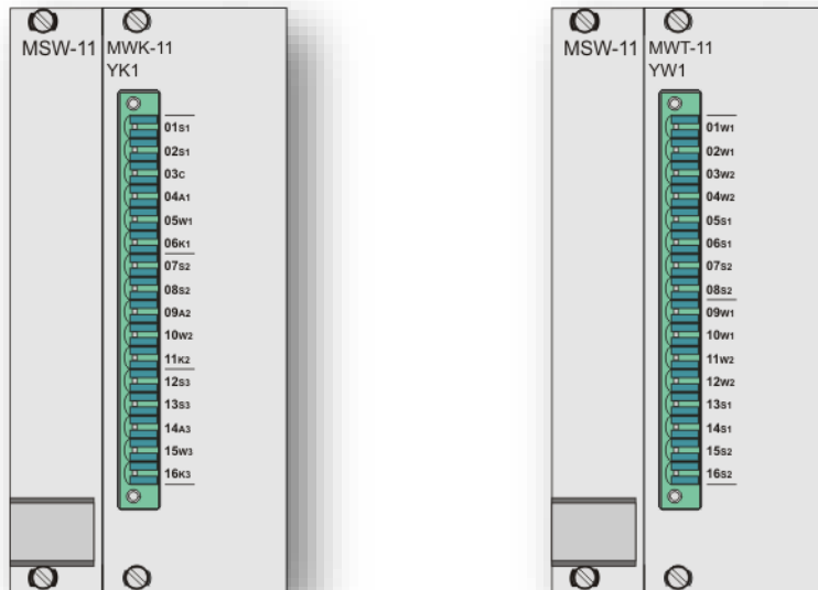
Rys. 5.26. Widok dostępnej dla użytkownika strony modułów wyłączników MF-11 i trójfazowych MW-11 wraz z modułem sterującym MSW-11.
