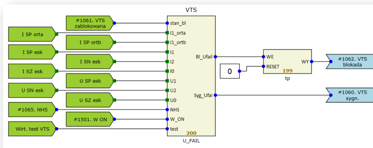
Rys. 7.26. Przykładowa konfiguracja funkcji VTS.
