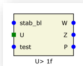
Rys. 7.17. Blok logiczny funkcji 59N U>1f.
