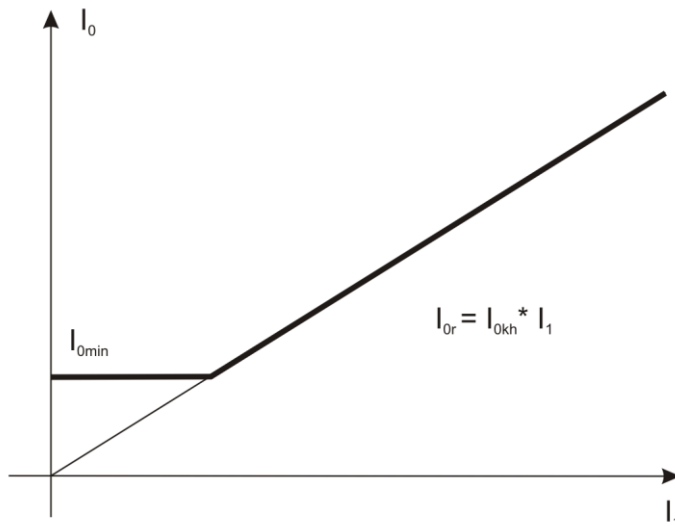
Rys. 7.23. Charakterystyka kryterium nadprądowego zerowego.
