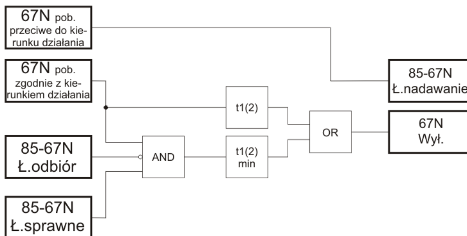
Rys. 7.10. Logika łącza w trybie blokującym.
