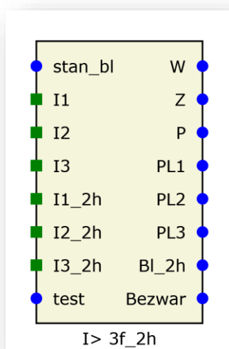
Rys. 7.11. Blok logiczny funkcji 50/51TD.
