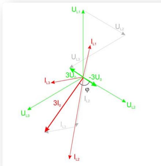
Rys. 7.2. Wykres wektorowy napięć i prądów – zwarcie na fazie L2 – kierunek „od szyn”.
