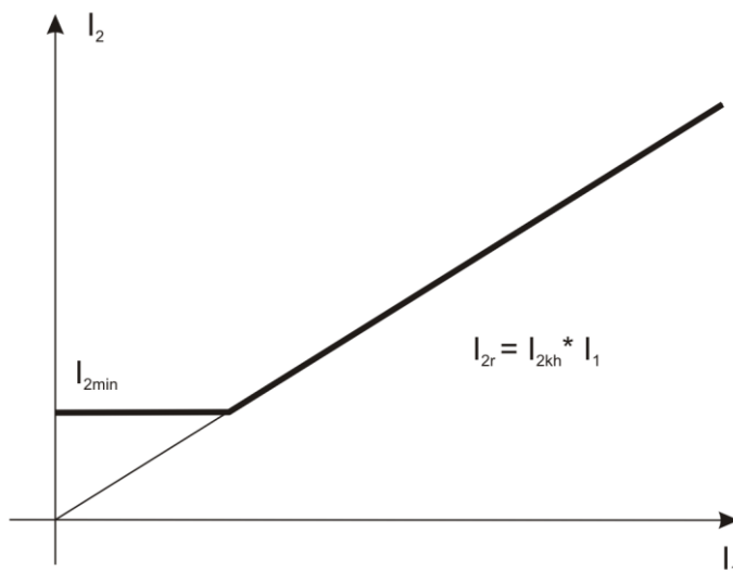
Rys. 7.24. Charakterystyka kryterium nadprądowego przeciwnego.
