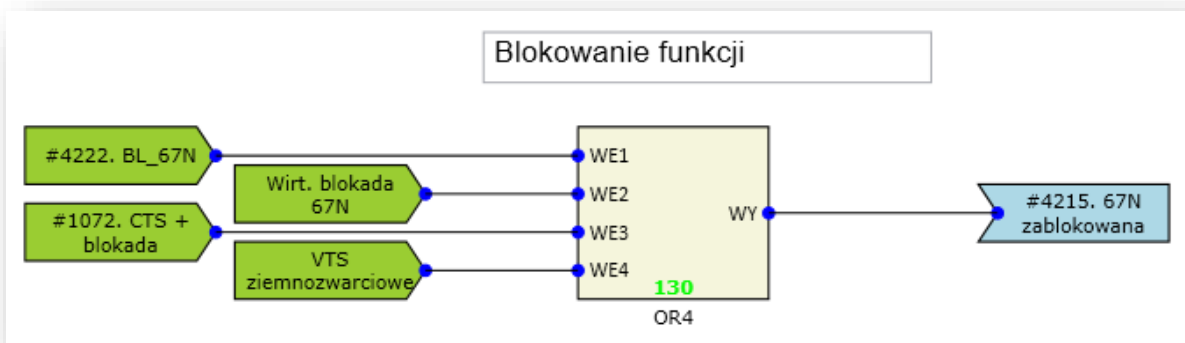
Rys. 7.8. Przykład realizacji blokady funkcji 67N.
