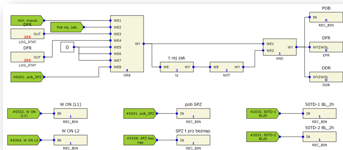
Rys. 7.33. Przykładowa konfiguracja funkcji DFR i DDR.
