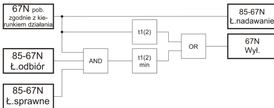
Rys. 7.9. Logika łącza w trybie zezwalającym.
