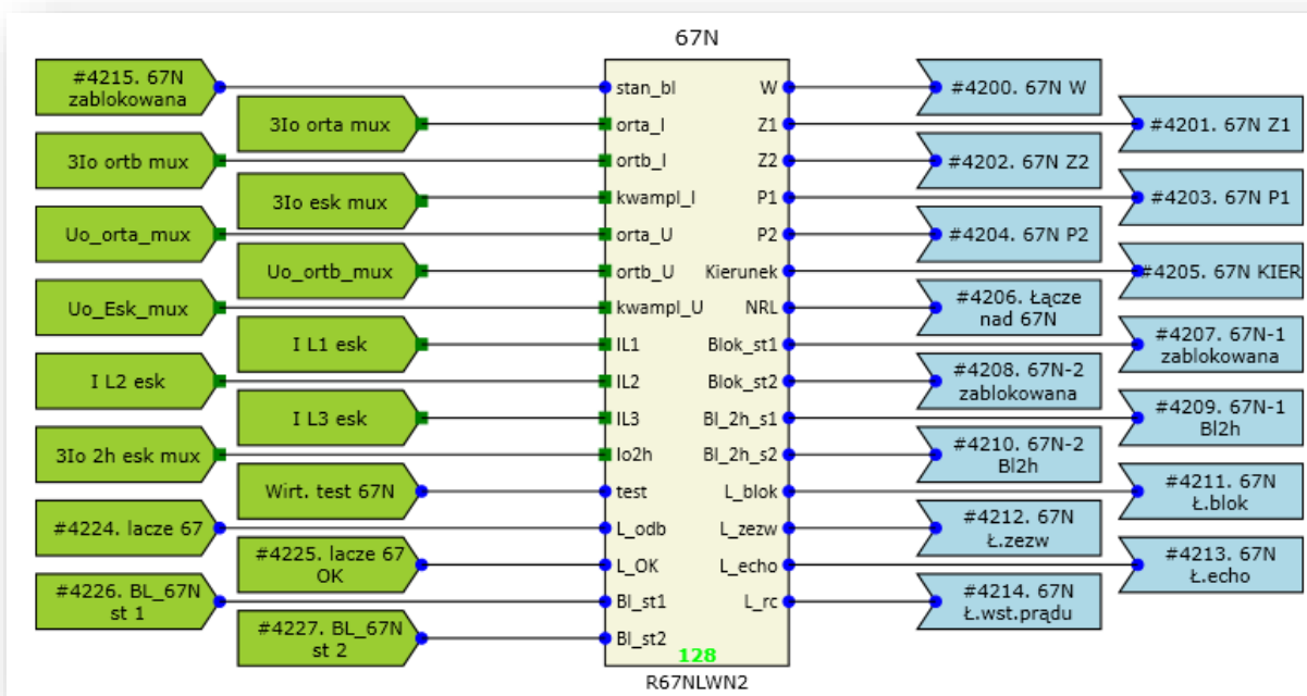
Rys. 7.7. Przykładowa konfiguracja funkcji R67N_LWN2 funkcji ziemnozwarciowej (67N).
