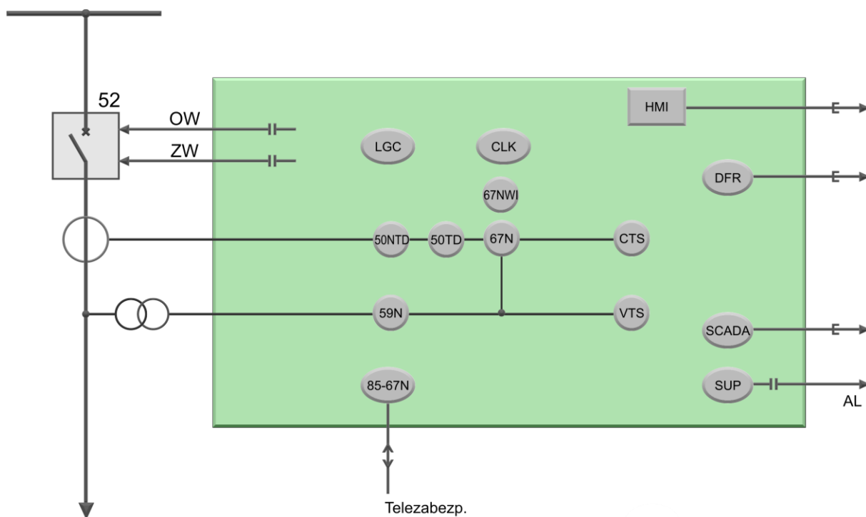
Rys. 3.1. Graficzne przedstawienie funkcji realizowanych przez urządzenie TZZ-11.
