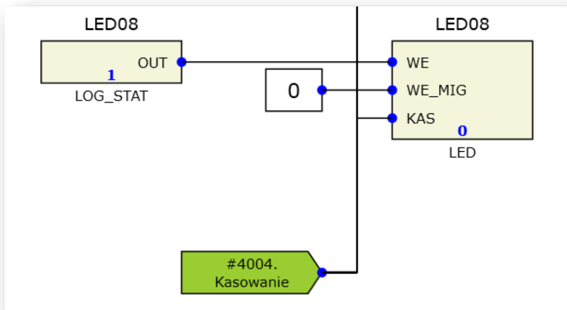
Rys. 7.42. Przykładowa konfiguracja funkcji LED.
