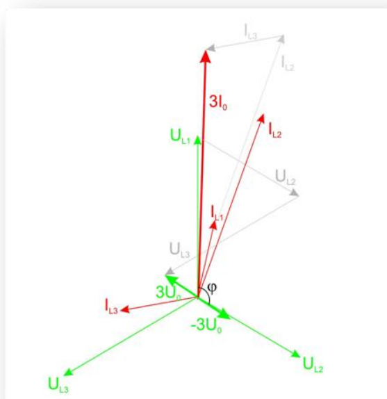
Rys. 7.3. Wykres wektorowy napięć i prądów – zwarcie na fazie L2 – kierunek „do szyn”.
