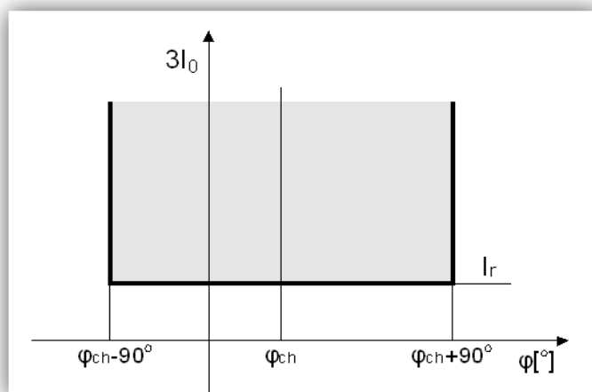
Rys. 7.5. Charakterystyka kątowna przekaźnika kierunkowego.
