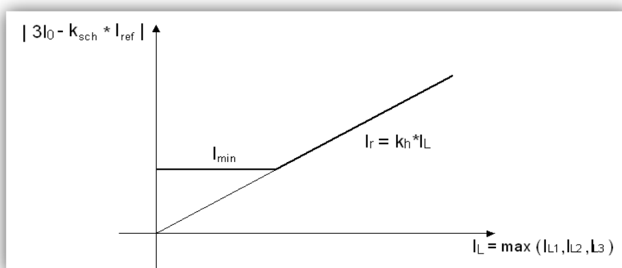
Rys. 7.28. Charakterystyka kryterium różnicowego.
