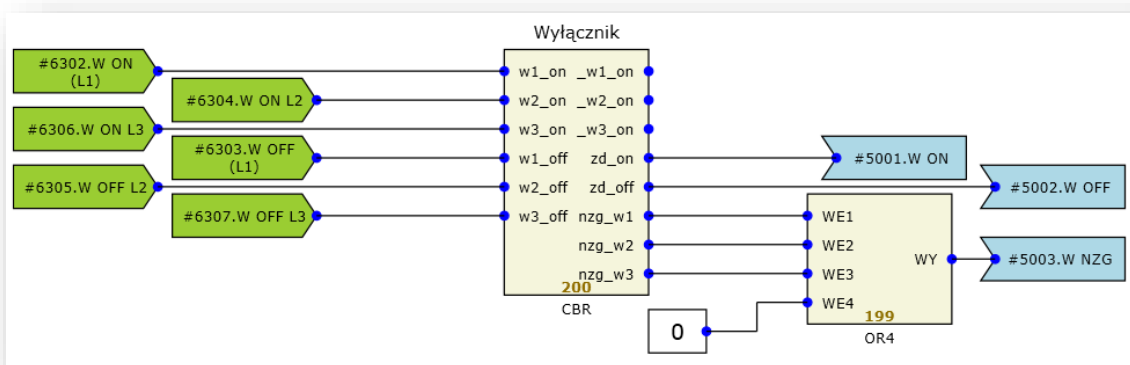
Rys. 7.21. Przykładowa konfiguracja funkcji CBR.
