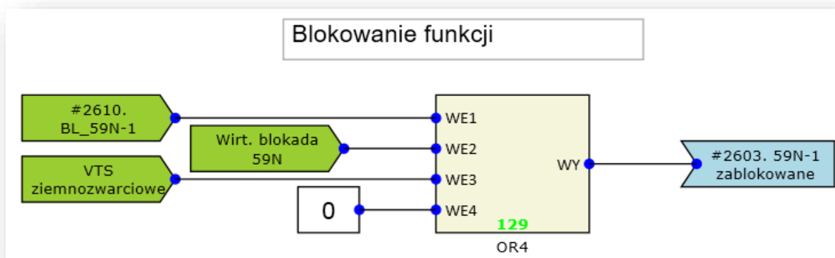
Rys. 7.19. Przykład realizacji blokady funkcji 59N.
