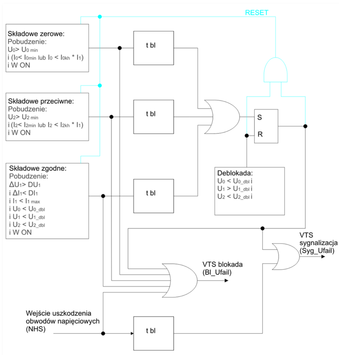
Rys. 7.22 Schemat blokowy działania funkcji VTS.
