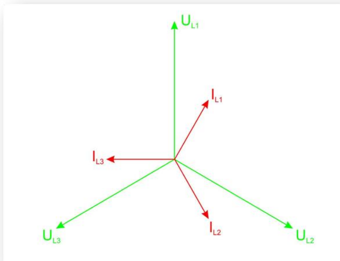
Rys. 7.1. Wykres wektorowy napięć i prądów – normalna praca.
