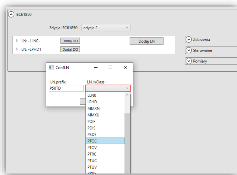
Rys. 7.51. Dodawanie węzłów.
