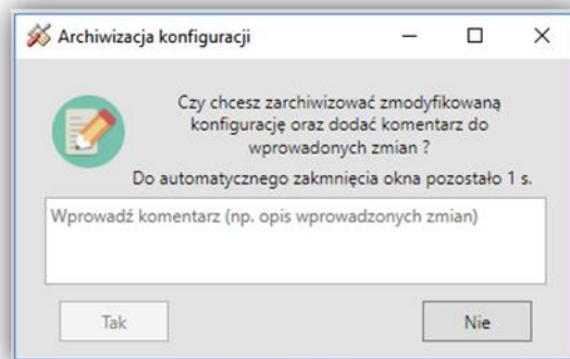
Rys. 9.68. Archiwizacja konfiguracji.
