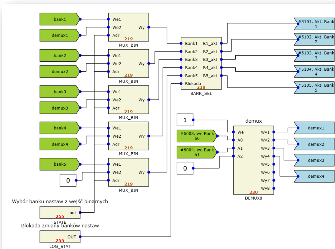
Rys. 7.44. Przykładowa konfiguracja wyboru banku nastaw.
