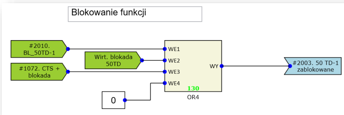
Rys. 7.13. Przykład realizacji blokady funkcji 50TD.
