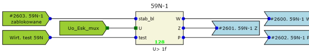
Rys. 7.18. Przykładowa konfiguracja funkcji 59N.
