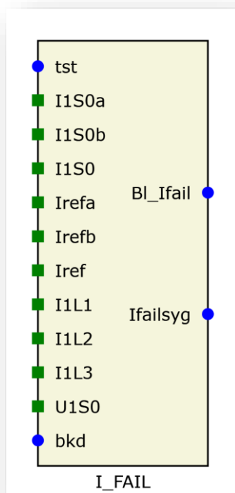
Rys. 7.29. Blok logiczny funkcji I_FAIL.
