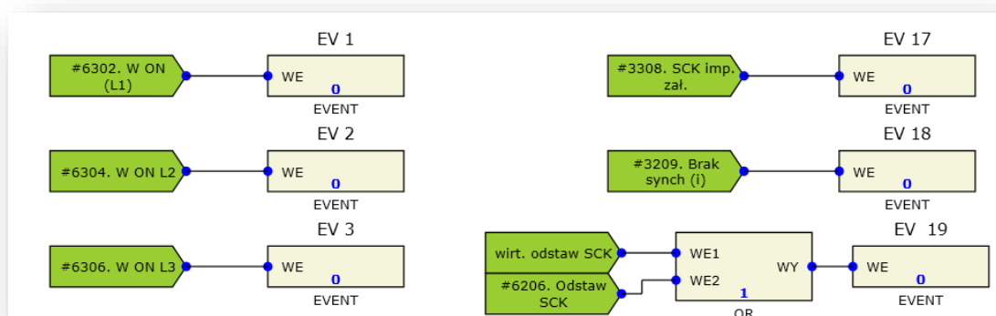
Rys. 7.37. Przykładowa konfiguracja funkcji rejestratora zdarzeń.
