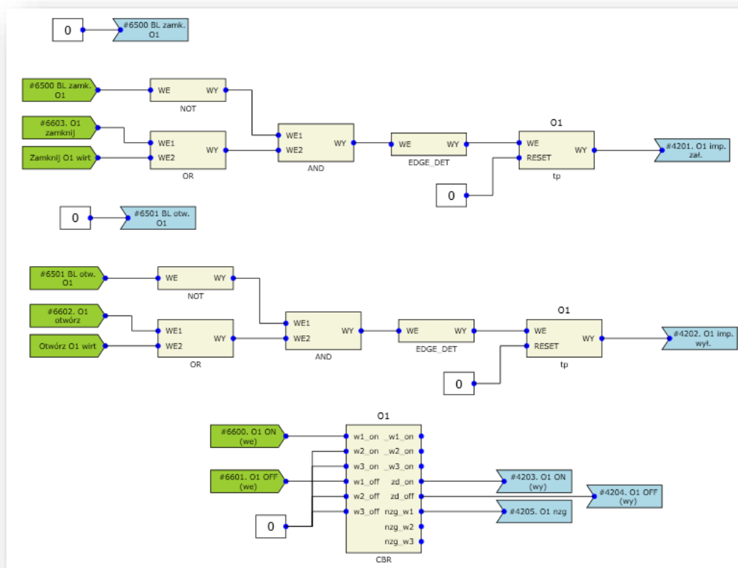
Rys. 7.38. Przykładowa konfiguracja sterownika polowego dla jednego łącznika.
