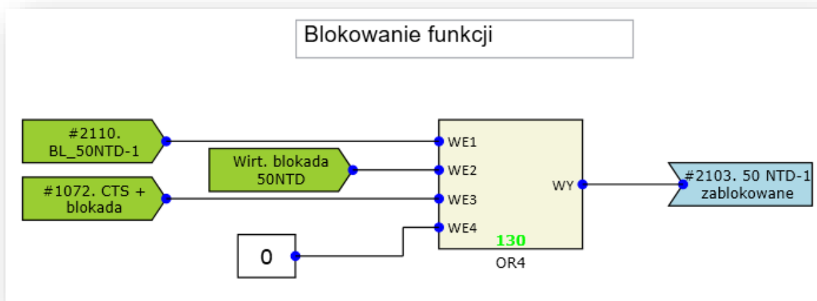
Rys. 7.16. Przykład realizacji blokady funkcji 50NTD.
