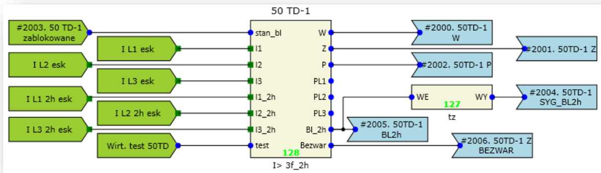
Rys. 7.12. Przykładowa konfiguracja funkcji 50TD.
