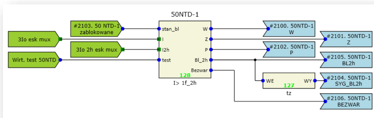
Rys. 7.15. Przykładowa konfiguracja funkcji 50NTD.
