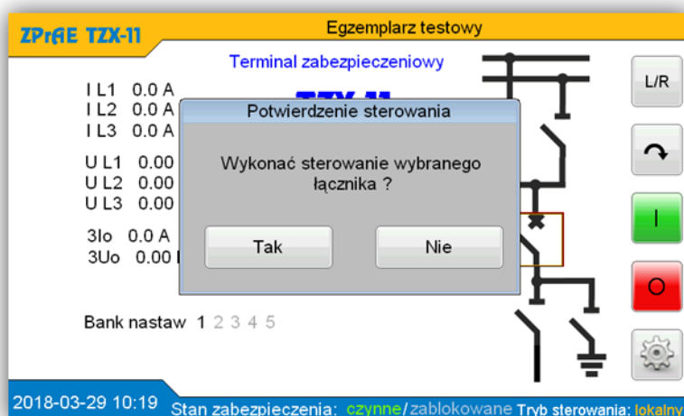
Rys. 6.5. Potwierdzenie sterowania.
