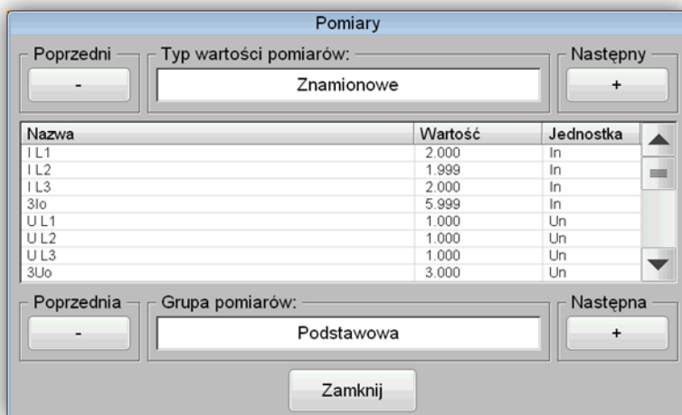
Rys. 6.15. Okno „Pomiary”.
