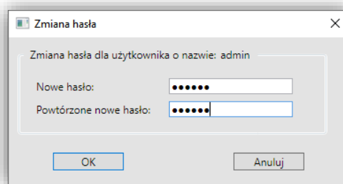
Rys. 9.21. Zmiana hasła.
