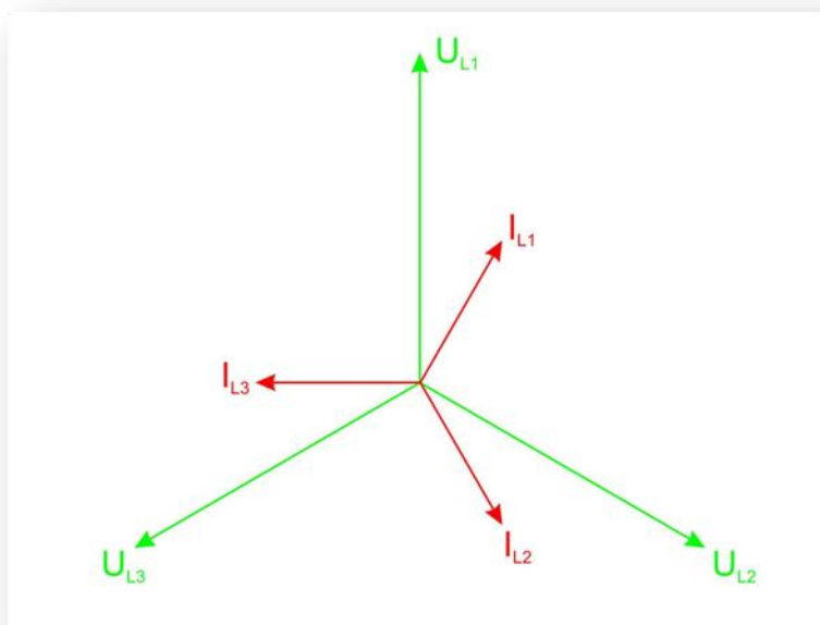
Rys. 7.34. Wykres wektorowy napięć i prądów – normalna praca.
