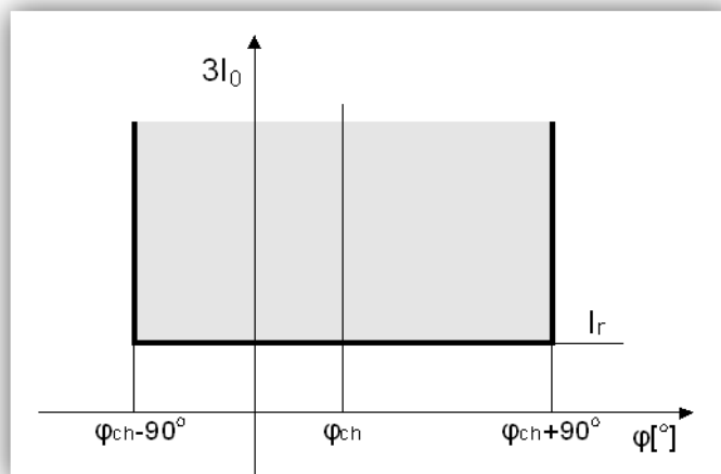
Rys. 7.38. Charakterystyka kątowa przełącznika kierunkowego.
