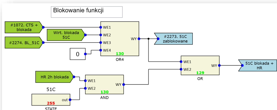
Rys. 7.6. Przykład realizacji blokady funkcji 51C.
