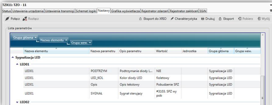
Rys. 7.65. Okno właściwości bloku LED w zakładce Nastawienia i opcji Sygnalizacja LED .
