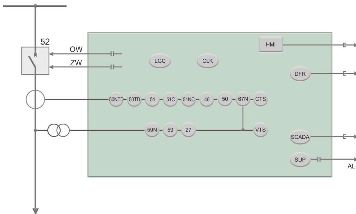
Rys. 3.1. Graficzne przedstawienie funkcji realizowanych przez urządzenie TZU-11.
