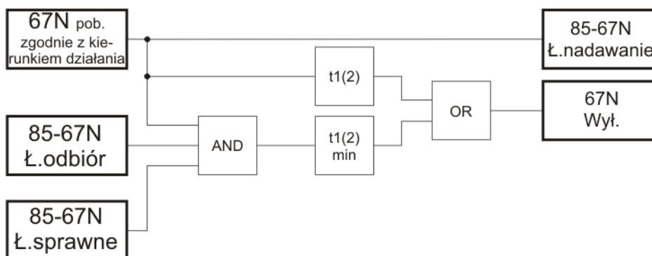
Rys. 7.42. Logika łącza w trybie zezwalającym.
