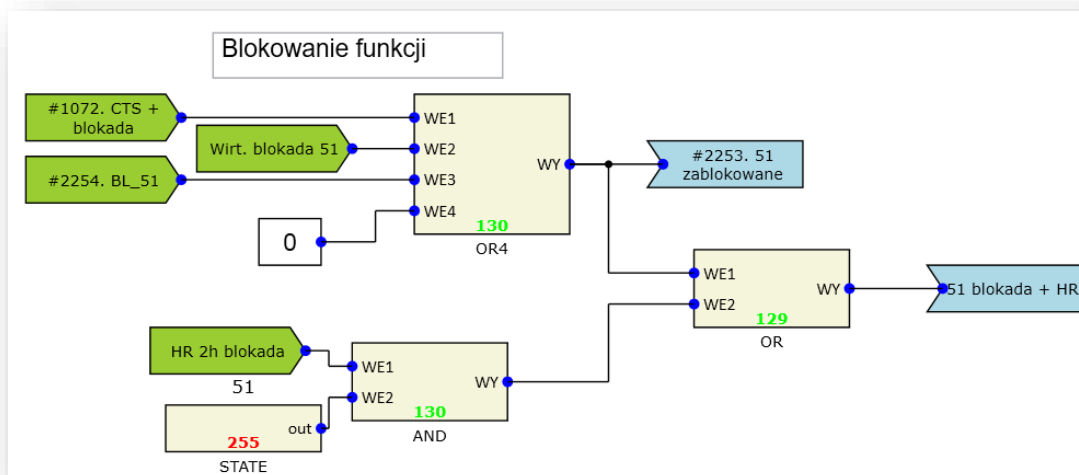
Rys. 7.5. Przykład realizacji blokady funkcji 51.
