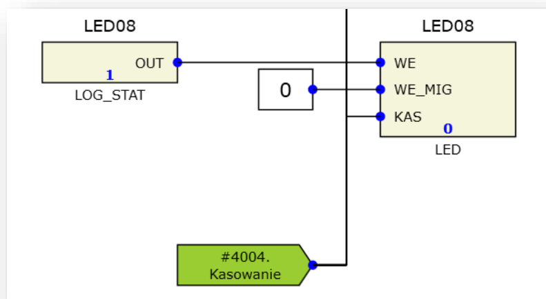
Rys. 7.67. Przykładowa konfiguracja funkcji LED.
