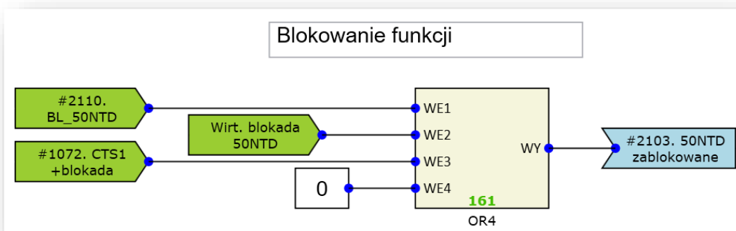
Rys. 7.19. Przykład realizacji blokady funkcji 50NTD.
