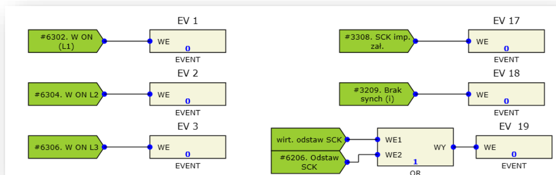
Rys. 7.63. Przykładowa konfiguracja funkcji rejestratora zdarzeń.
