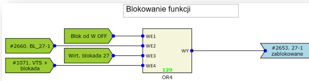
Rys. 7.33. Przykład realizacji blokady funkcji 27.
