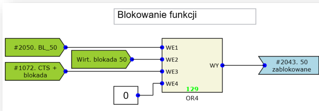
Rys. 7.16. Przykład realizacji blokady funkcji 50.
