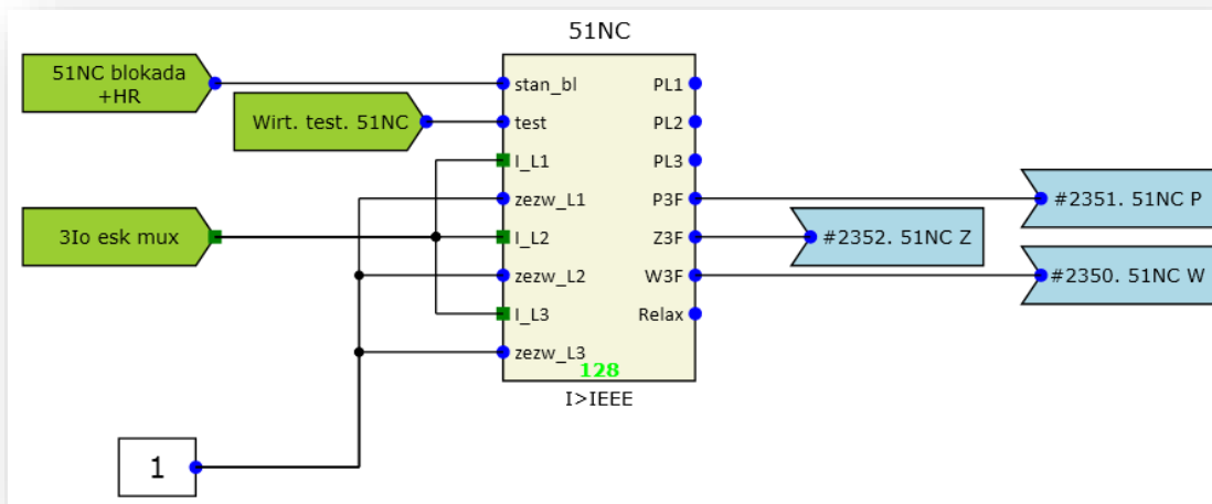
Rys. 7.10. Przykładowa konfiguracja funkcji nadprądowej ziemnozwarciowej zależnej 51NC.
