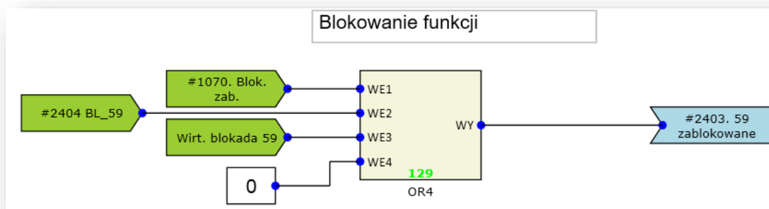
Rys. 7.29. Przykład realizacji blokady funkcji 59.
