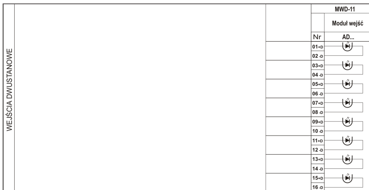
Rys. 5.3. Schemat połączeń modułu wejść dwustanowych MWD-11.
