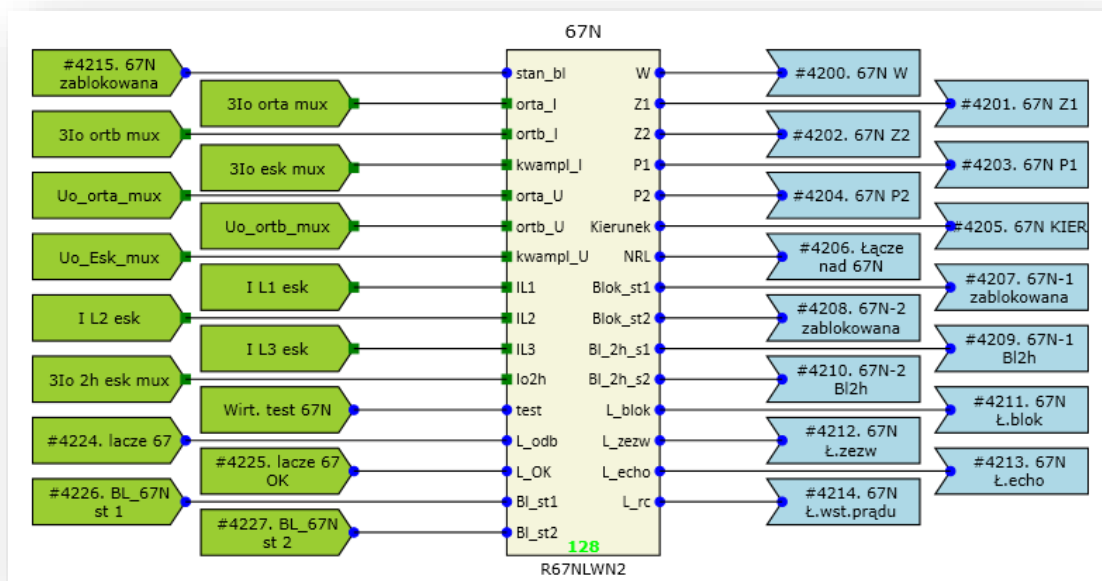
Rys. 7.40. Przykładowa konfiguracja funkcji R67N_LWN2 funkcji ziemnozwarciowej (67N).
