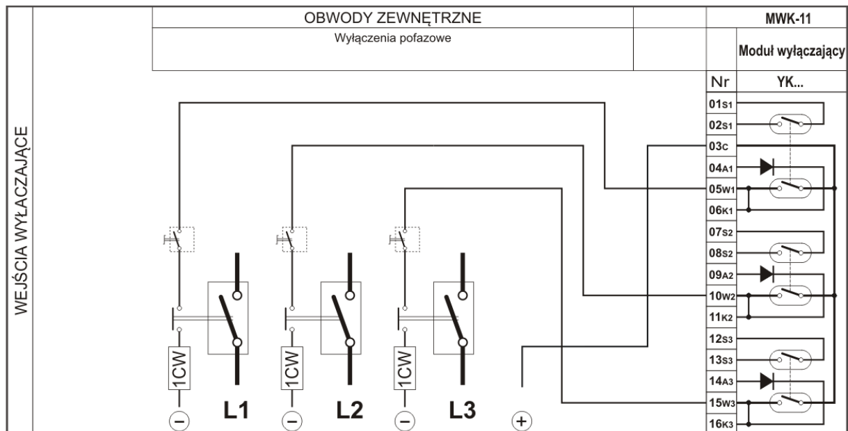
Rys. 5.24. Moduł przekaźników wyłączających szybkich-mocnych dla układów wyłączeń pofazowych.
