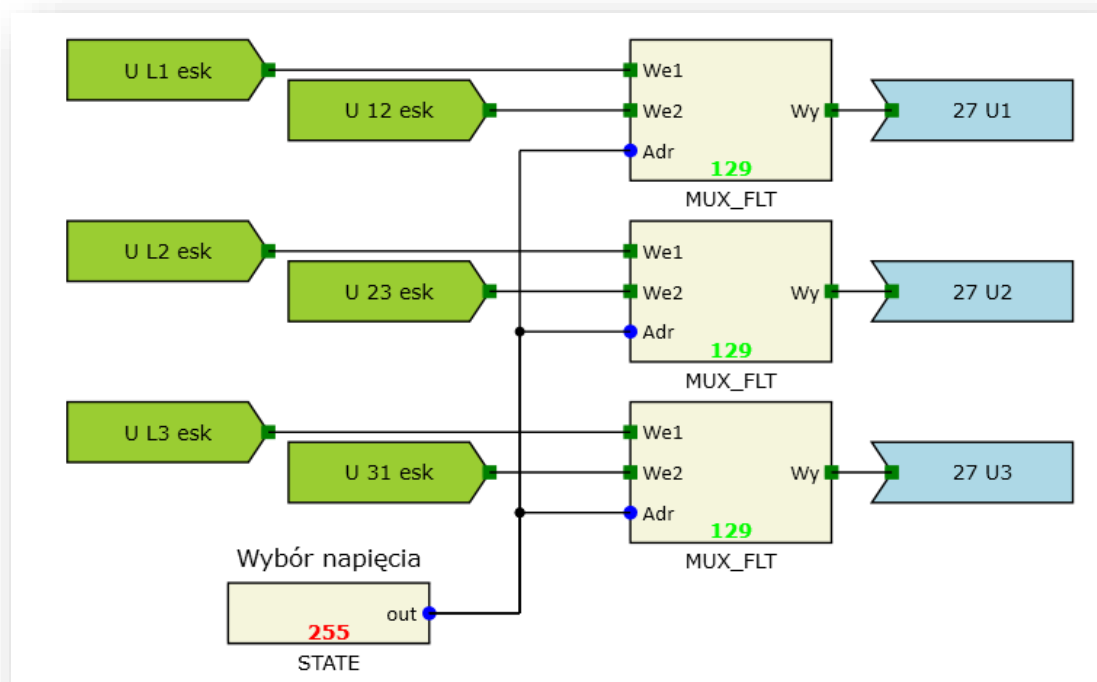
Rys. 7.31. Przykładowa konfiguracja funkcji 27.
