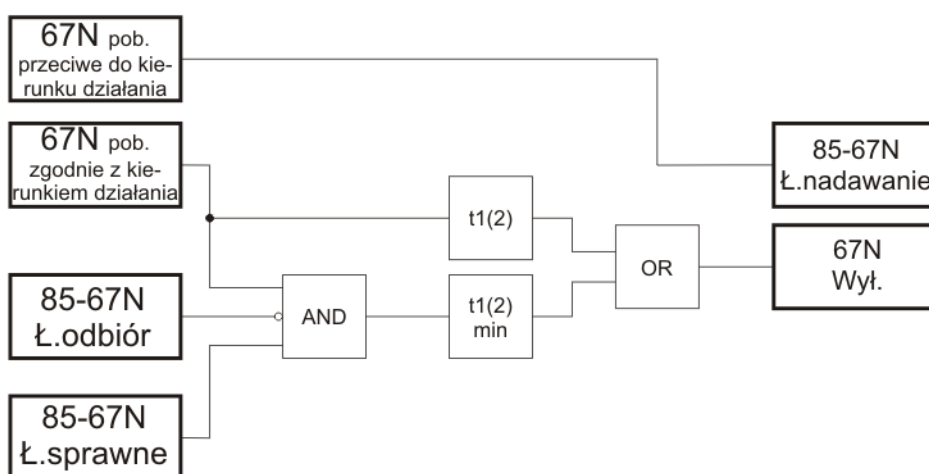
Rys. 7.43. Logika łącza w trybie blokującym.
