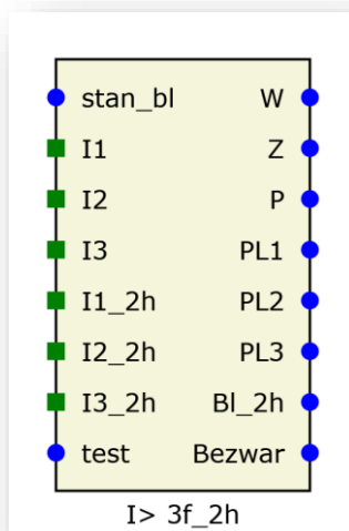
Rys. 7.12. Blok logiczny funkcji 51/50TD.
