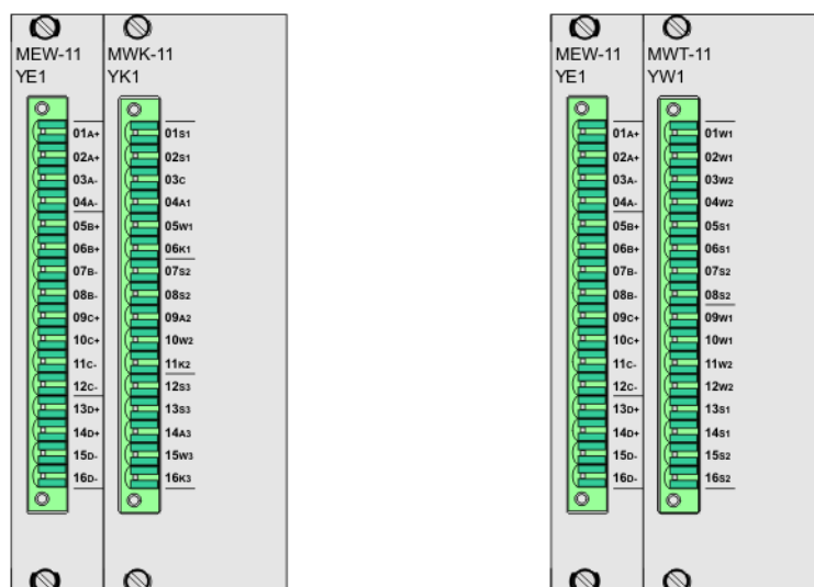
Rys. 5.30. Zastosowanie MEW-11 jako modułu sterującego dla modułu wyłączników pofazowych MKW-11 i trójfazowych MWT-11.
