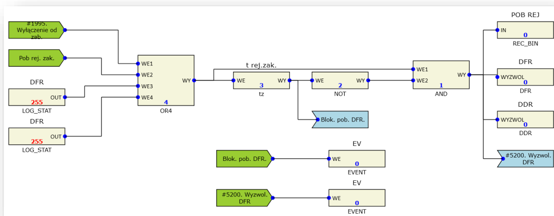
Rys. 7.59. Przykładowa konfiguracja funkcji DFR i DDR.
