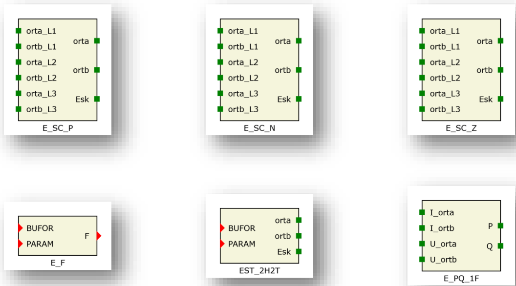
Rys. 9.46. Bloki logiczne dla grupy „estymaty”.
