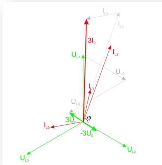
Rys. 7.36. Wykres wektorowy napięć i prądów – zwarcie na fazie L2 – kierunek „do szyn”.
