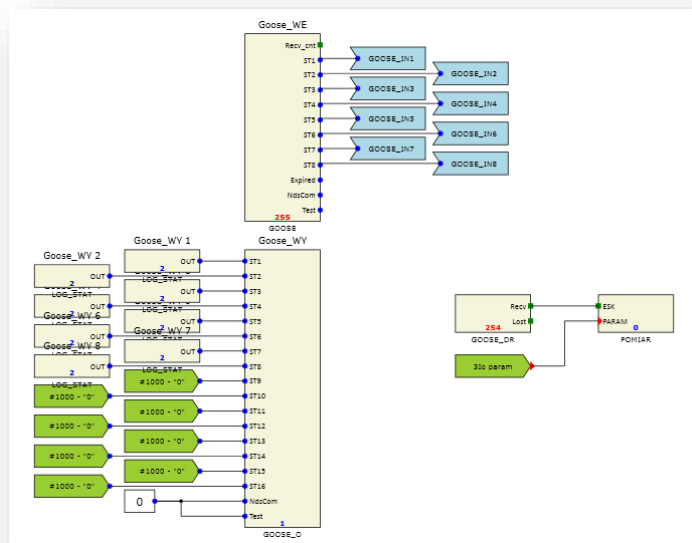
Rys. 7.72. Schemat funkcji odbierania i wysyłania komunikatów GOOSE.
