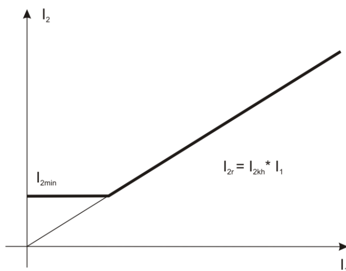
Rys. 7.50. Charakterystyka kryterium nadprądowego przeciwnego.
