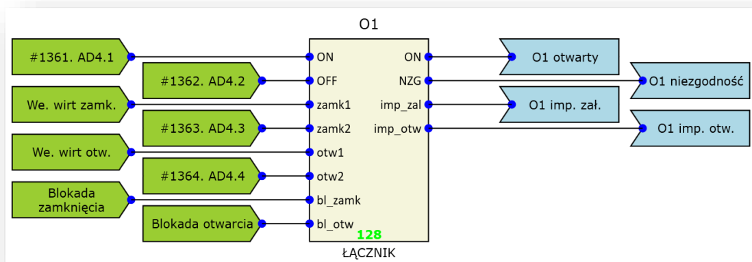
Rys. 7.71. Przykładowa konfiguracja pojedynczego łącznika.
