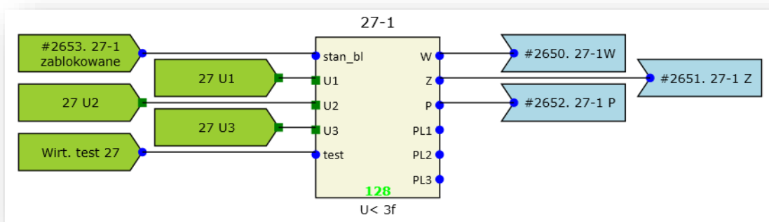
Rys. 7.31. Przykładowa konfiguracja funkcji 27.
