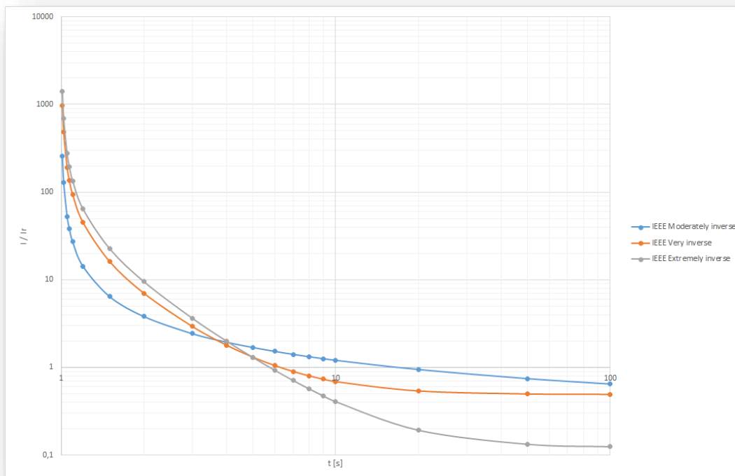
Rys. 7.8. Charakterystyki czasowe IDMT predefiniowane.
