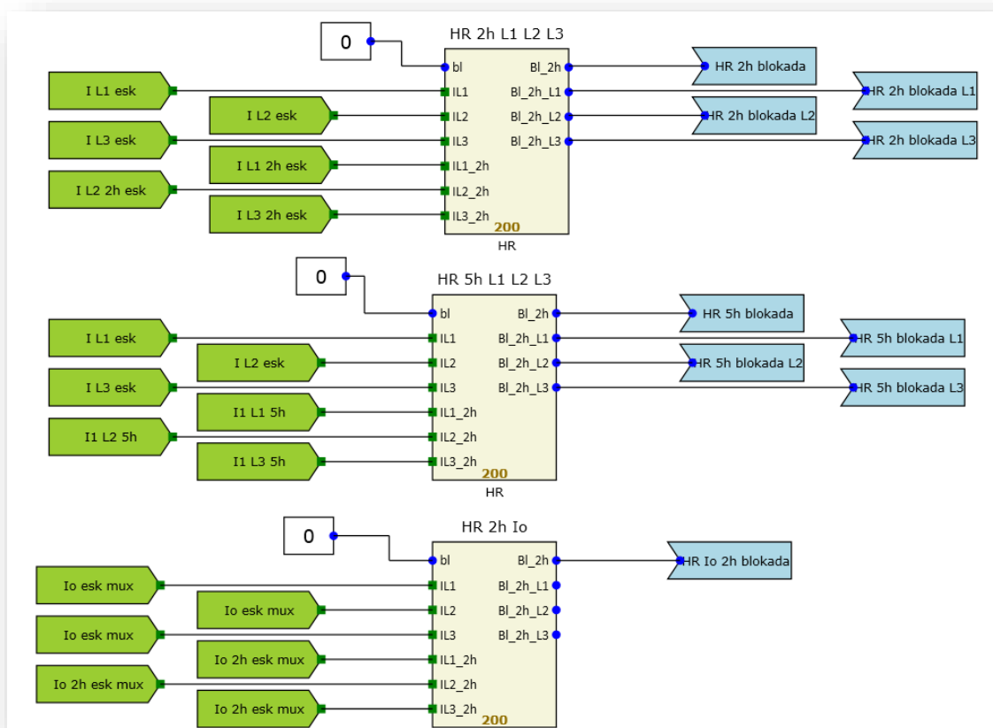
Rys. 7.45. Przykładowa konfiguracja funkcji HR.
