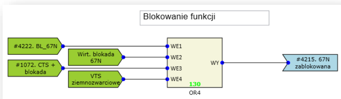
Rys. 7.41. Przykład realizacji blokady funkcji 67N.
