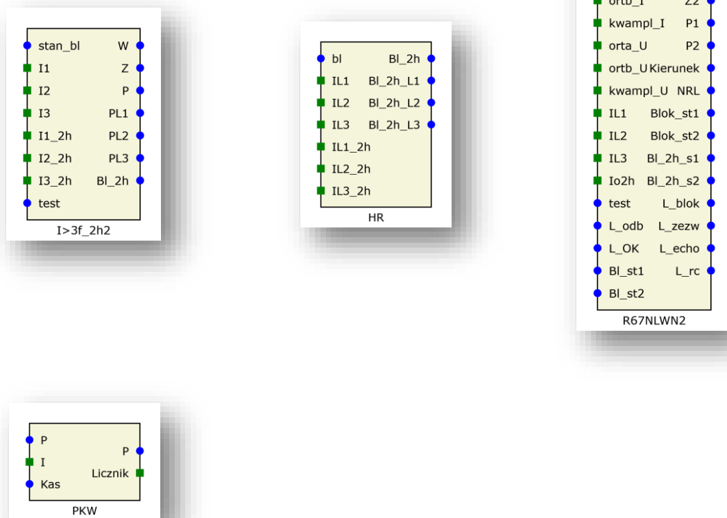
Rys. 9.49. Bloki logiczne dla grupy „f.zabezpieczeniowe” cz. 2.
