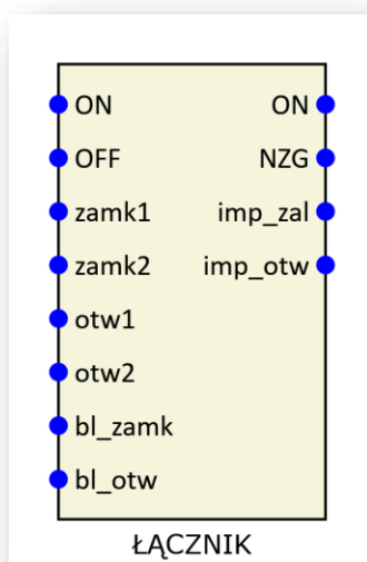
Rys. 7.70. Blok logiczny funkcji ŁACZNIK.
