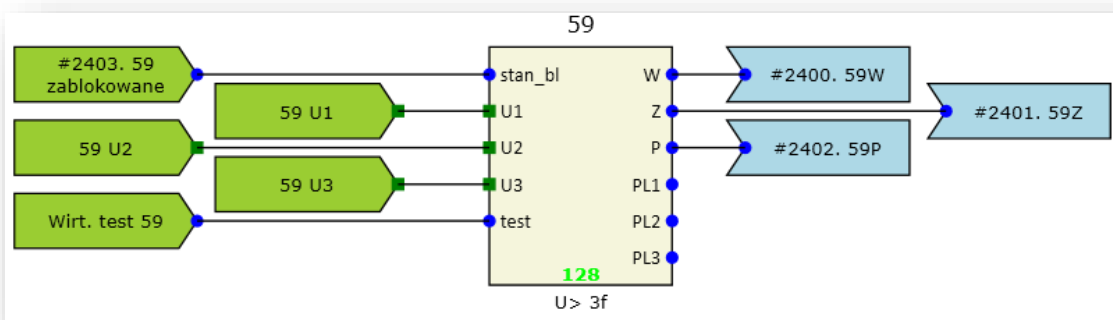
Rys. 7.27. Przykładowa konfiguracja funkcji 59.
