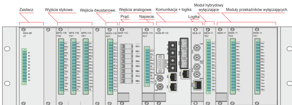
Rys. 4.6. Rozmieszczenie złączy dla przykładowego zabezpieczenia TZU-11.
