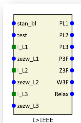
Rys. 7.3. Blok logiczny I>IEEE funkcji nadprądowej zależnej (51).
