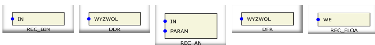
Rys. 7.58. Bloki logiczne związane z funkcjami DFR i DDR.
