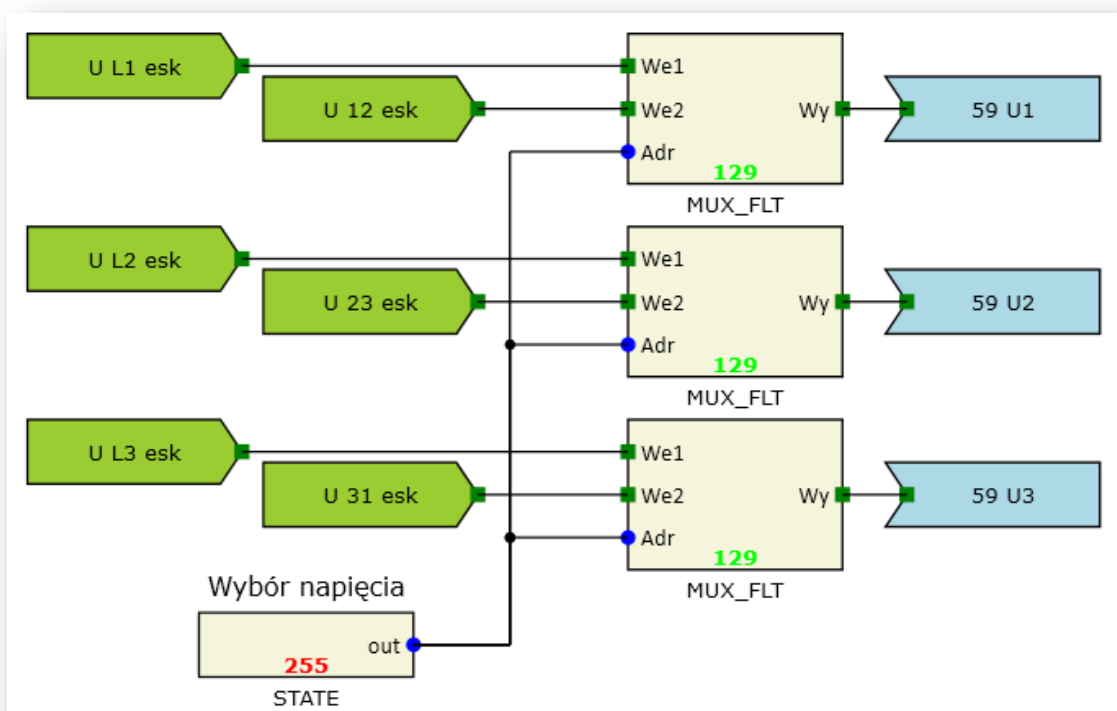
Rys. 7.27. Przykładowa konfiguracja funkcji 59.
