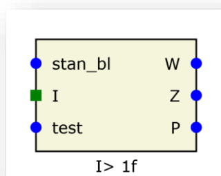
Rys. 7.20. Blok logiczny funkcji 46 wykorzystujący funkcję I > 1f .
