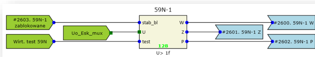
Rys. 7.24. Przykładowa konfiguracja funkcji 59N.
