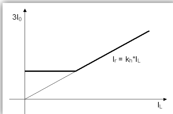
Rys. 7.37. Charakterystyka działania członu naprądowego zerowego stabilizowanego.
