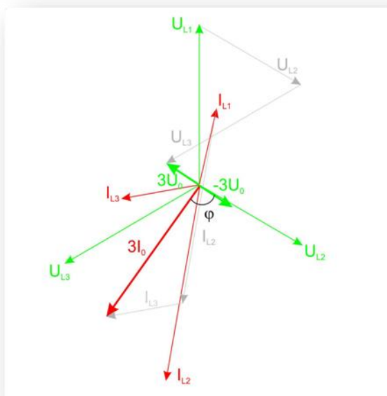
Rys. 7.35. Wykres wektorowy napięć i prądów – zwarcie na fazie L2 – kierunek „od szyn”.
