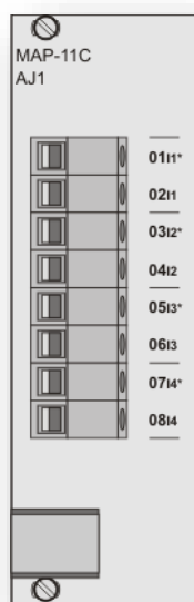
Rys. 5.13. Moduł analogowy prądowy.
