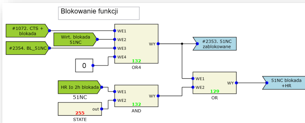
Rys. 7.11. Przykład realizacji blokady funkcji 51NC.
