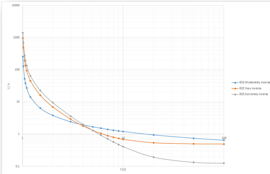
Rys. 7.2. Charakterystyki czasowe IDMT predefiniowane.
