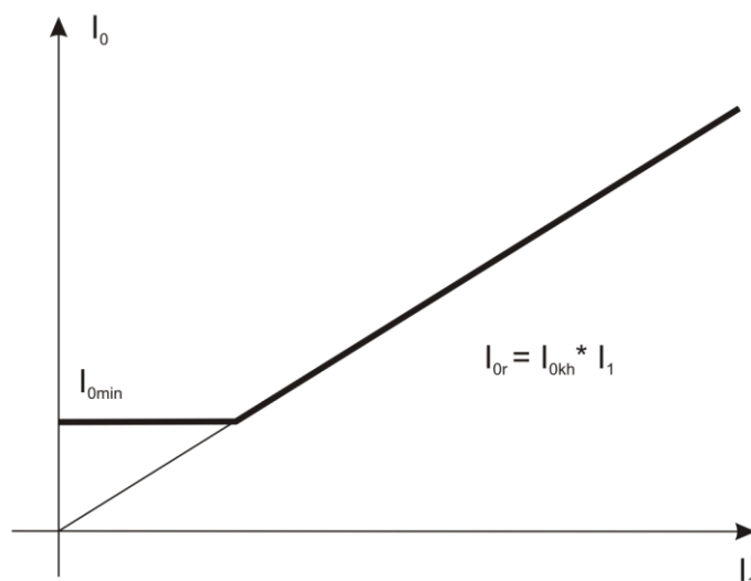
Rys. 7.49. Charakterystyka kryterium nadprądowego zerowego.
