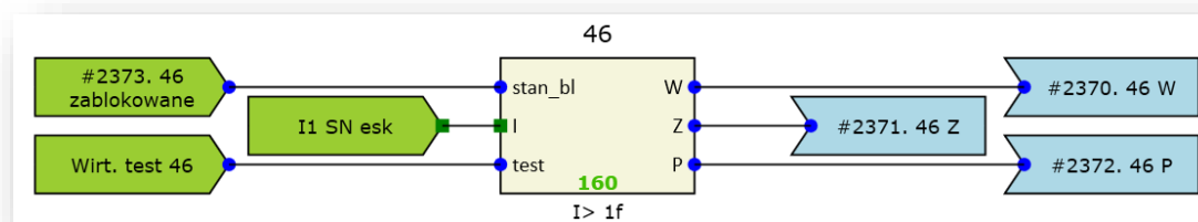
Rys. 7.21. Przykładowa konfiguracja funkcji 46.
