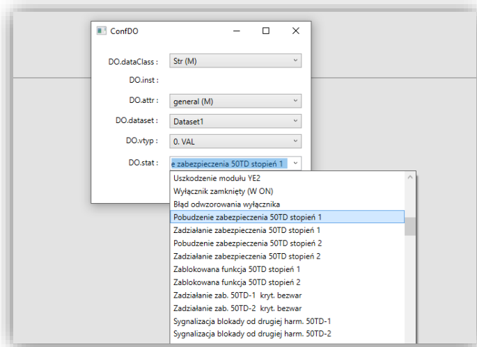
Rys. 7.81. Przypisywanie zdarzeń do atrybutu danej.
