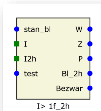
Rys. 7.17. Blok logiczny funkcji 51/50NTD.
