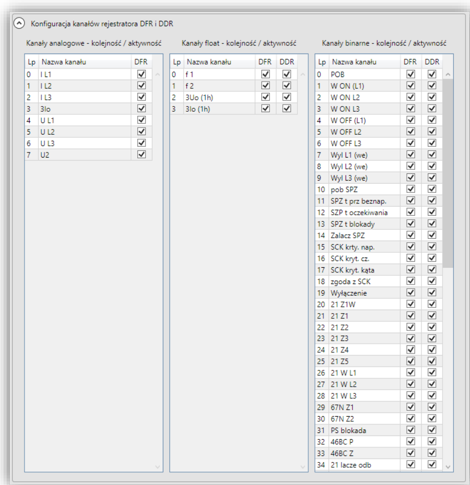
Rys. 9.80. Konfiguracja kanałów rejestratora DFR i DDR.
