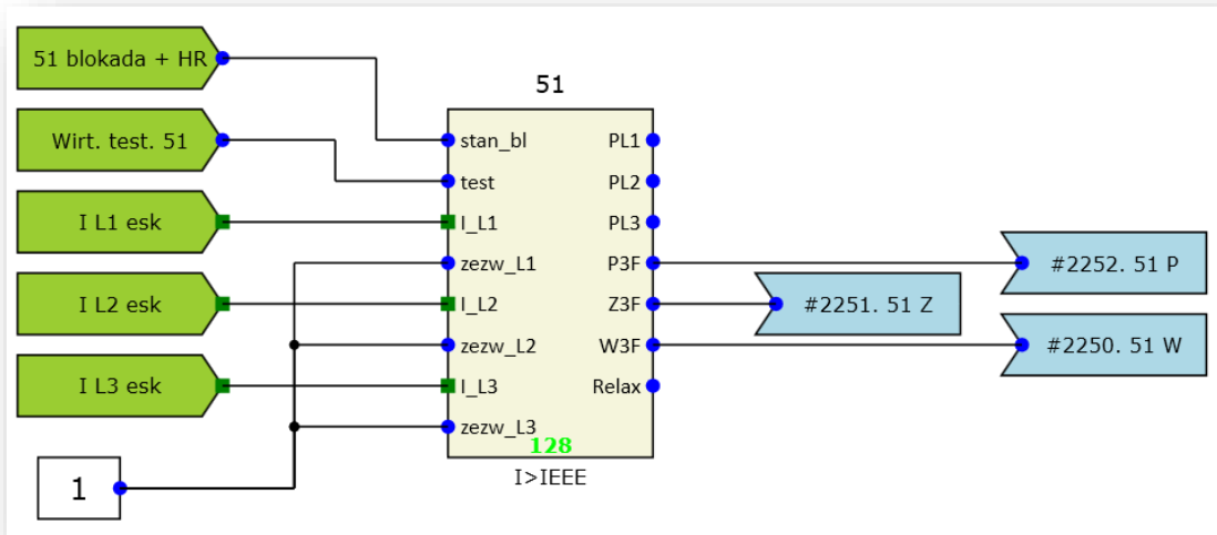
Rys. 7.4. Przykładowa konfiguracja funkcji nadprądowej zależnej 51.
