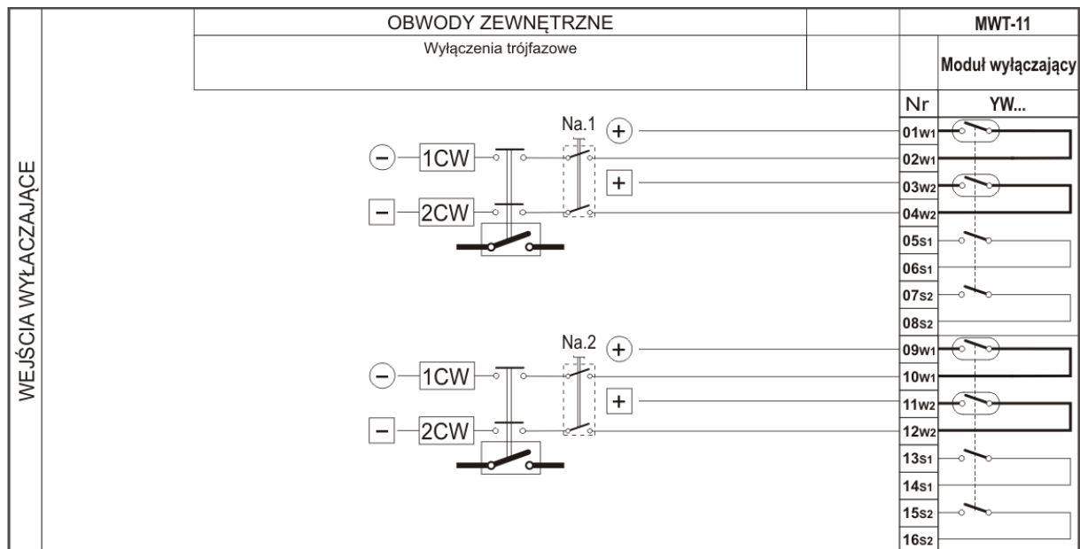
Rys. 5.25. Moduł przekaźników wyłączających szybkich-mocnych dla układów wyłączeń trójfazowych.
