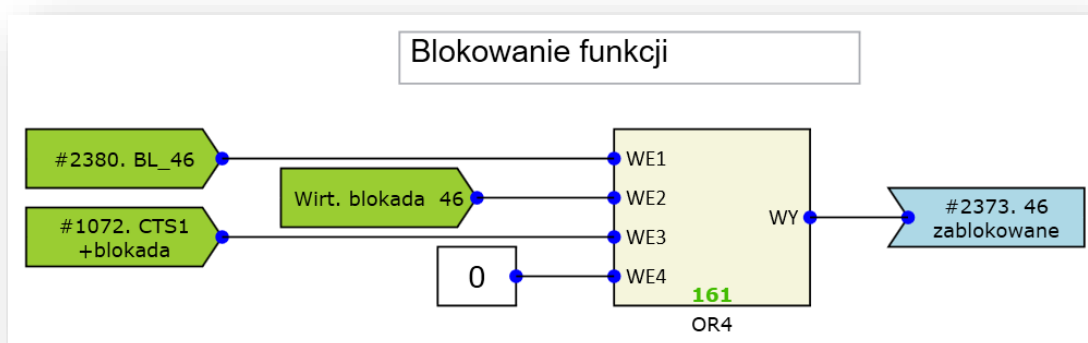
Rys. 7.22. Przykład realizacji blokady funkcji 46.
