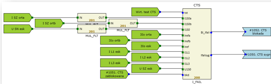
Rys. 7.56. Przykładowa konfiguracja funkcji CTS.
