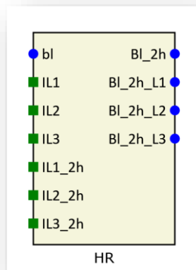
Rys. 7.44. Blok logiczny funkcji HR.
