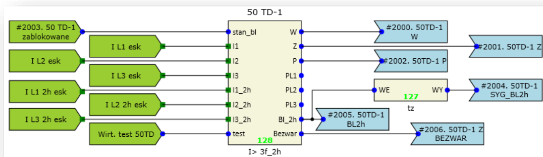
Rys. 7.13. Przykładowa konfiguracja funkcji 50TD.
