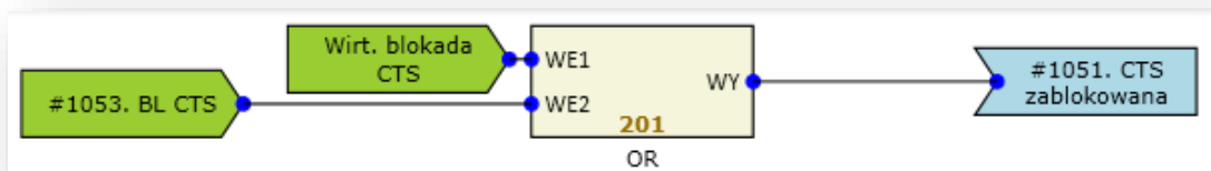
Rys. 7.57. Przykład realizacji blokady funkcji CTS.
