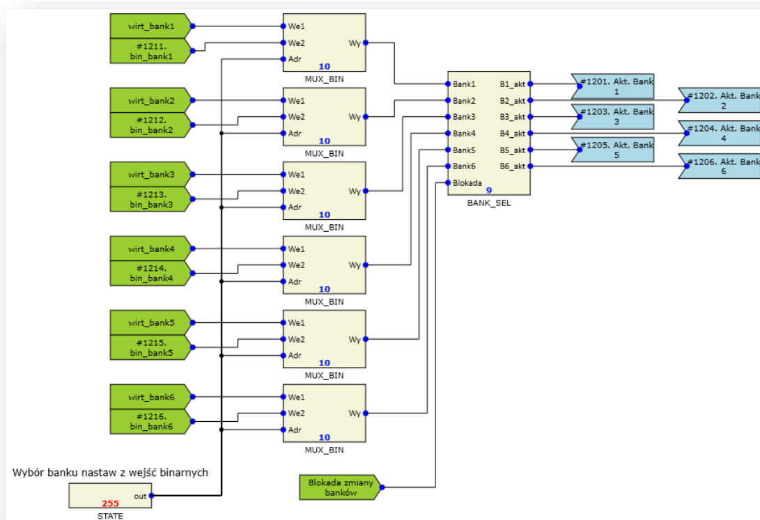
Rys. 7.69. Przykładowa konfiguracja wyboru banku nastaw.
