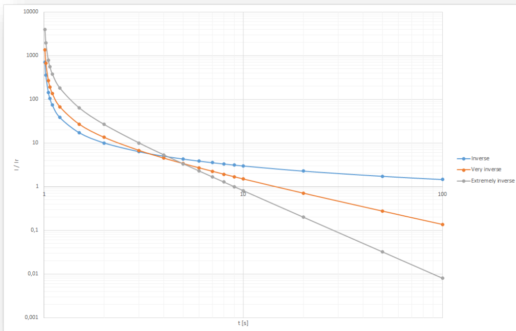
Rys. 7.7. Charakterystyki czasowe zależne predefiniowane.
