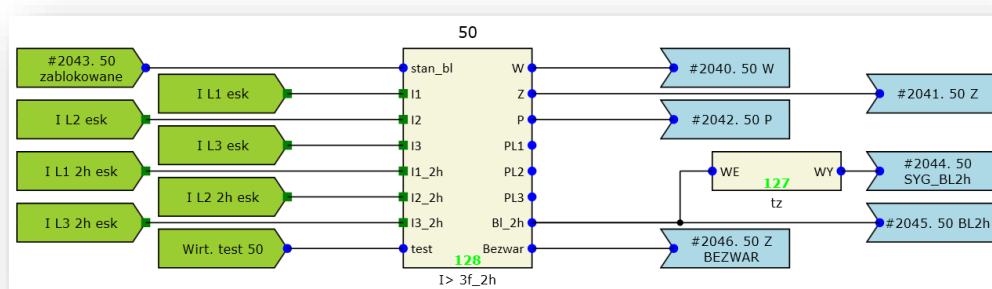
Rys. 7.15. Przykładowa konfiguracja funkcji 50.
