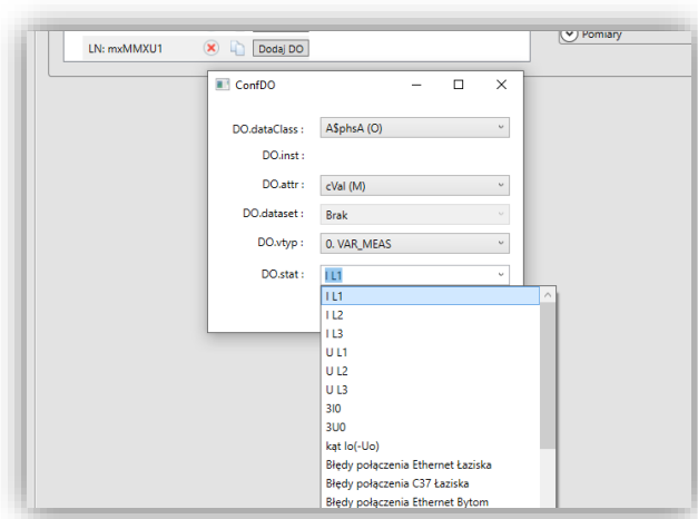
Rys. 7.84. Konfiguracja pomiaru. Wybór pomiaru: prąd faza L1.
