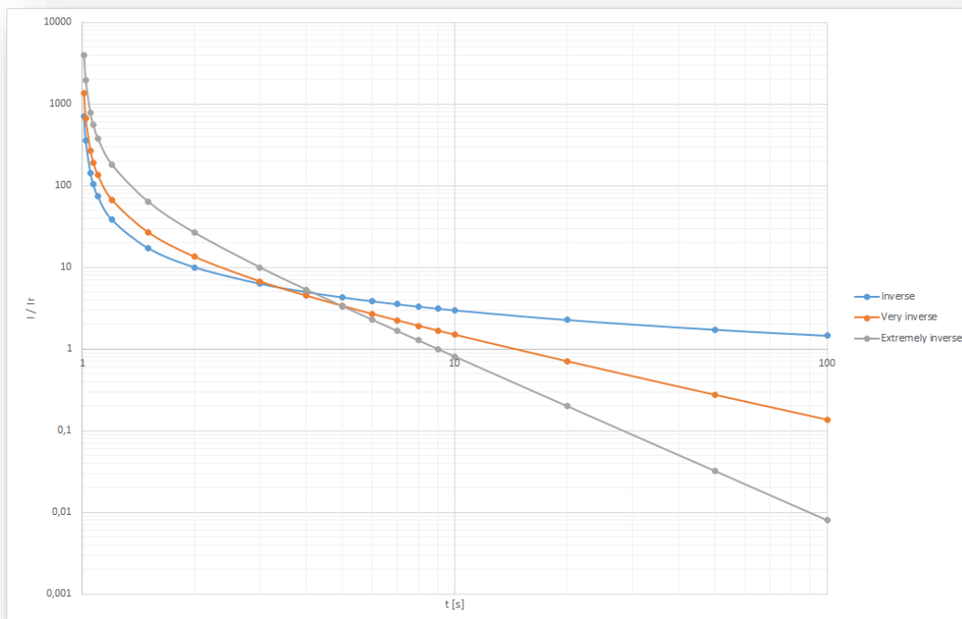
Rys. 7.1. Charakterystyki czasowe zależne predefiniowane.
