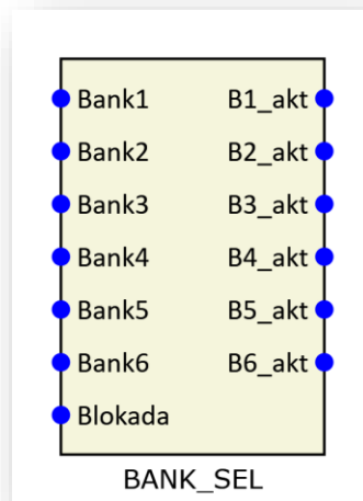
Rys. 7.68. Blok logiczny BANK_SEL.
