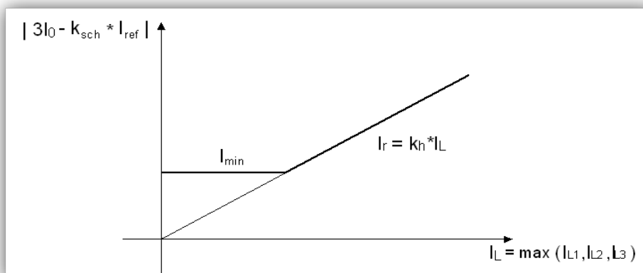
Rys. 7.32. Charakterystyka kryterium różnicowego.
