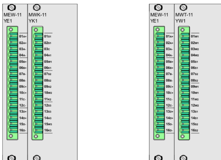
Rys. 5.30. Zastosowanie MEW-11 jako modułu sterującego dla modułu wyłączń pofazowych MKW-11 i trójfazowych MWT-11.
