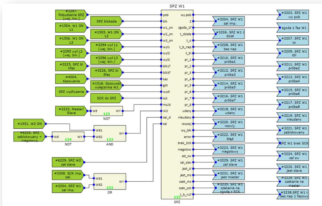
Rys. 7.4. Przykładowa konfiguracja funkcji SPZ (79).
