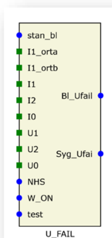
Rys. 7.29. Blok logiczny funkcji U_FAIL .
