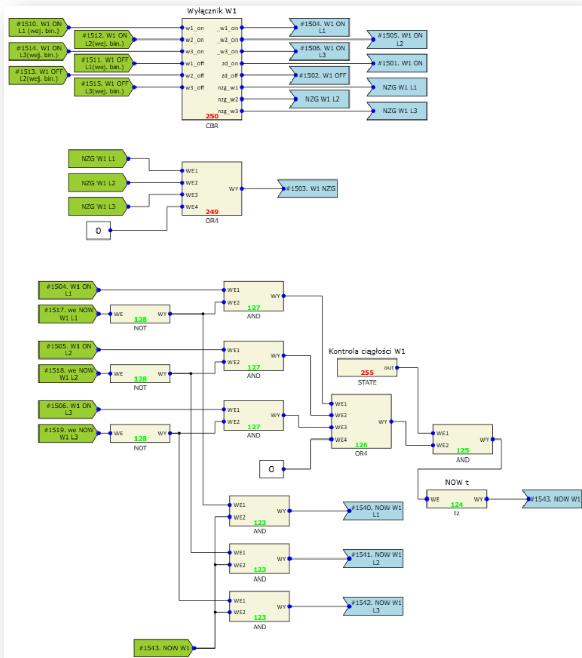
Rys. 7.20. Przykładowa konfiguracja funkcji CBR.
