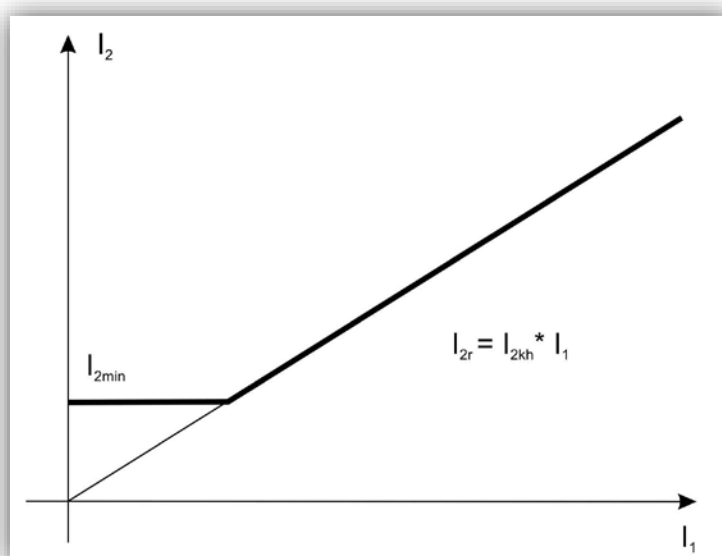
Rys. 7.28. Charakterystyka kryterium nadprądowego przeciwnego.
