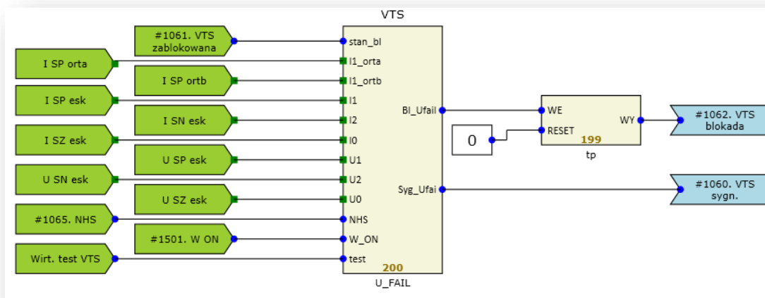
Rys. 7.30. Przykładowa konfiguracja funkcji VTS.
