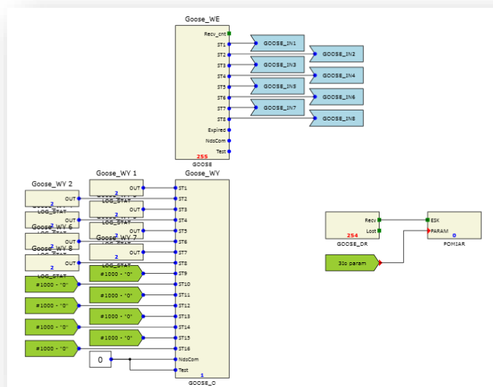
Rys. 7.36. Schemat funkcji odbierania i wysyłania komunikatów GOOSE.
