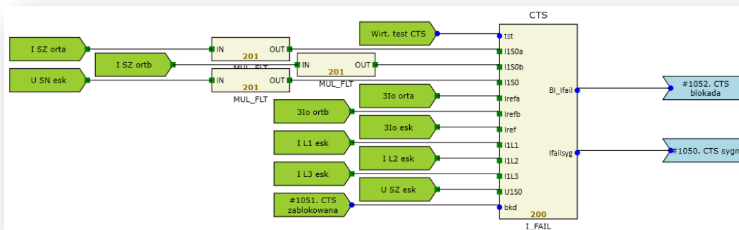
Rys. 7.34. Przykładowa konfiguracja funkcji CTS.
