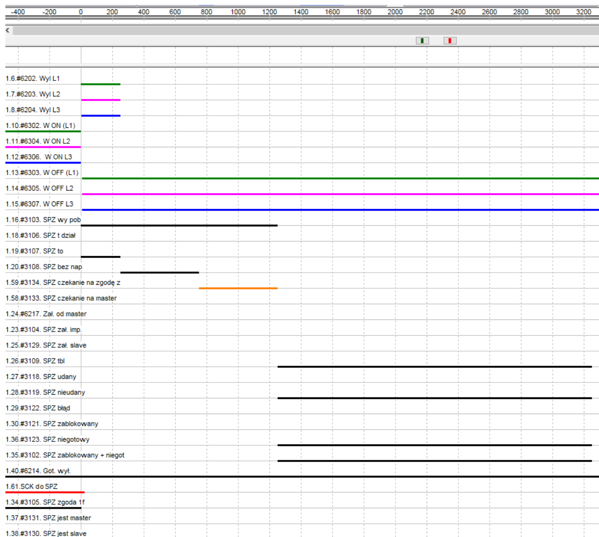
Rys. 7.13. Nieudany SPZ z powodu braku zgody z układu kontroli synchronizmu
