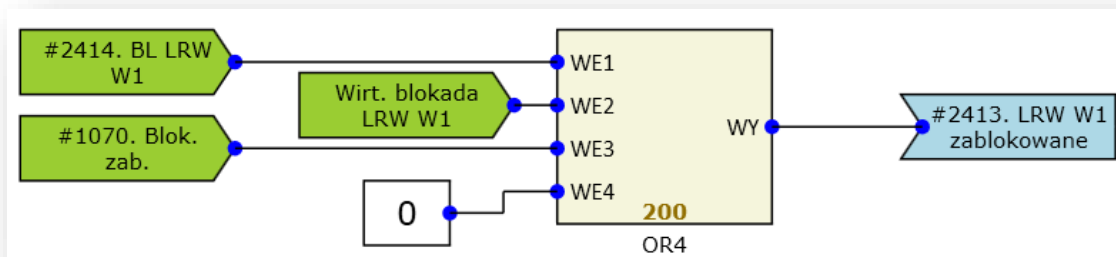
Rys. 7.23. Przykład realizacji blokady funkcji LRW.
