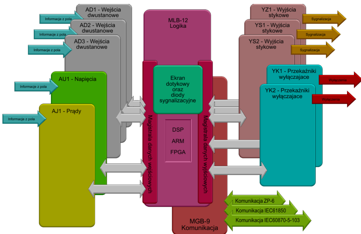
Rys. 2.1. Schemat blokowy pokazujący budowę urządzenia zabezpieczeniowego TZS-11.
