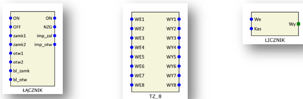
Rys. 9.44. Bloki logiczne dla grupy „Logika” c.d.
