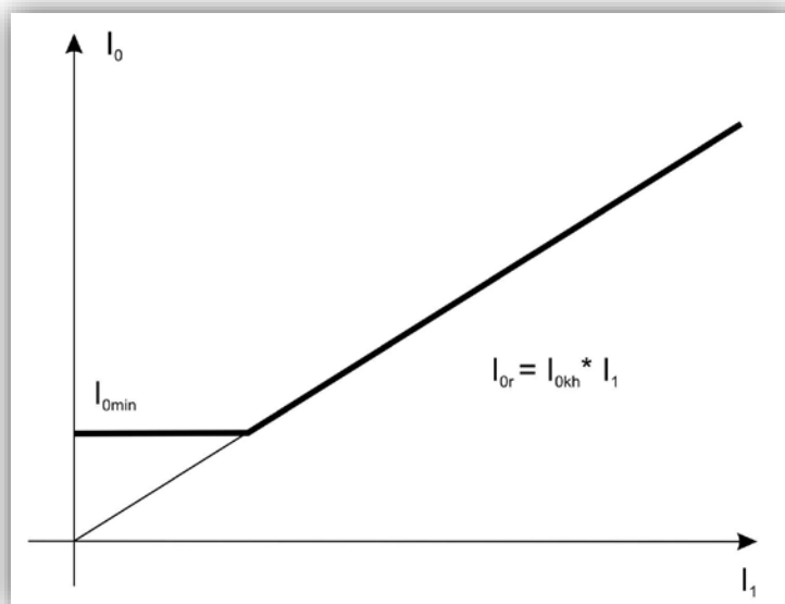
Rys. 7.27. Charakterystyka kryterium nadprądowego zerowego.
