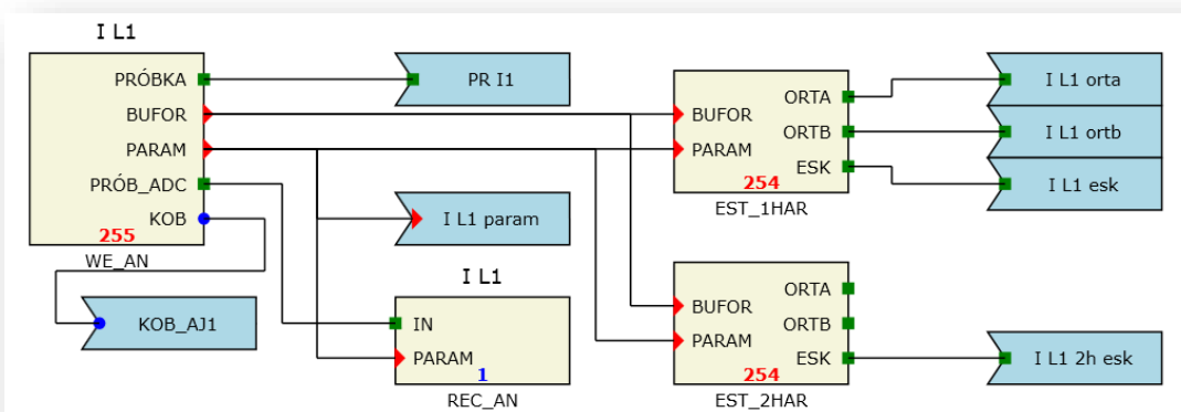
Rys. 5.18. Przykładowa konfiguracja wejścia prądowego.
