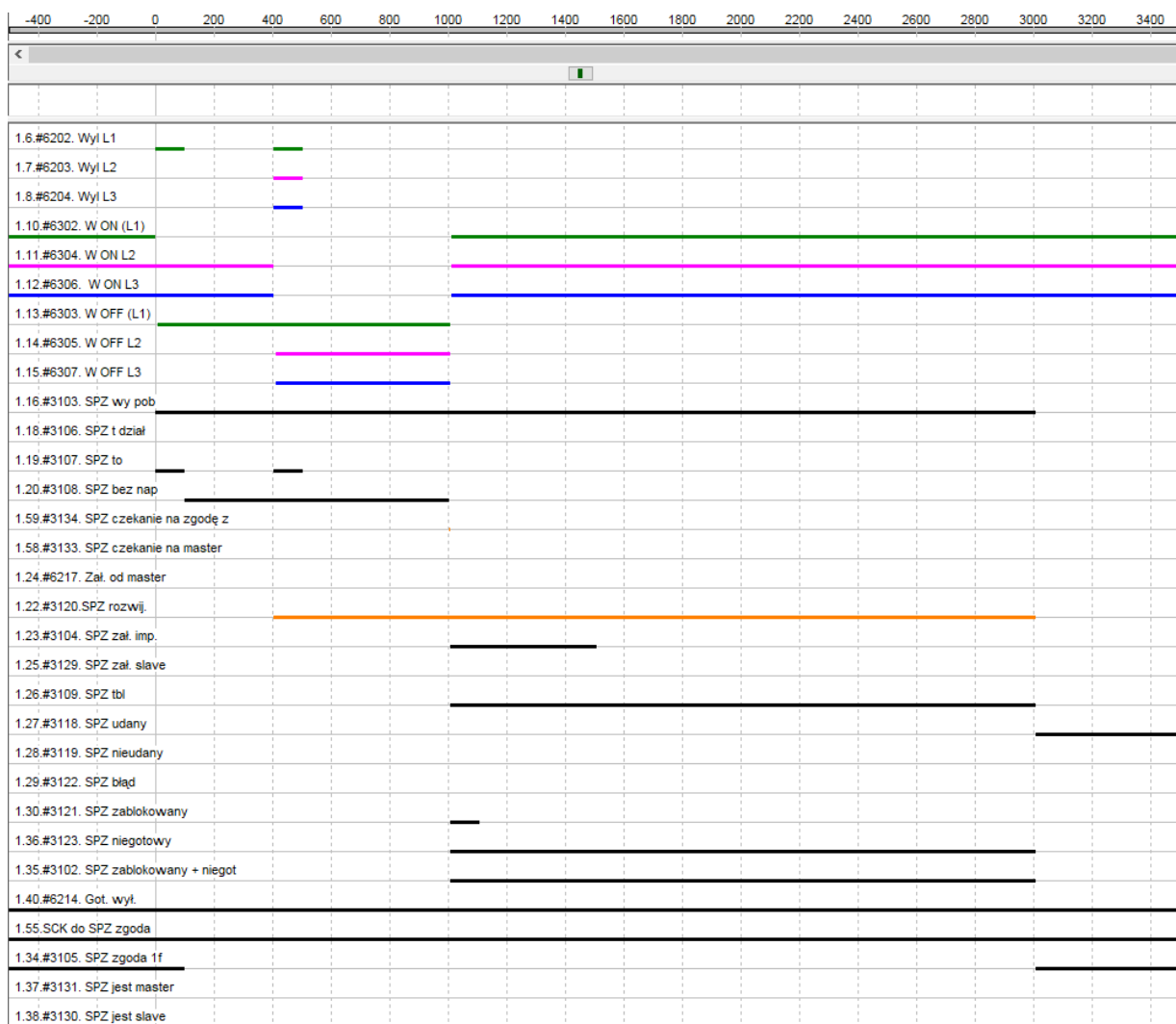
Rys. 7.10. Zwarcie rozwijające się.
