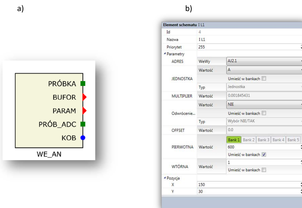
Rys. 5.15. Blok wejścia analogowego wraz z oknem właściwości a) blok wejścia analogowego WE_AN, b) właściwości bloku WE_AN.
