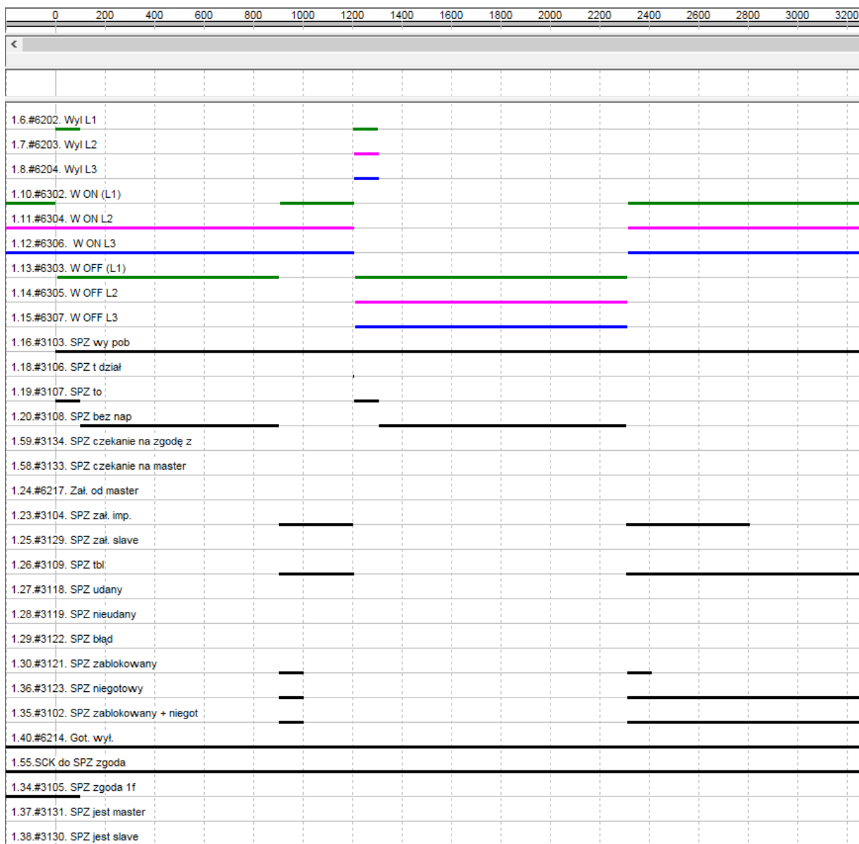
Rys. 7.9. SPZ 1 i 3- fazowy
