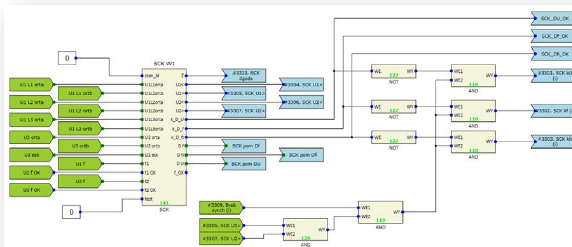
Rys. 7.17. Przykładowa konfiguracja funkcji SCK .
