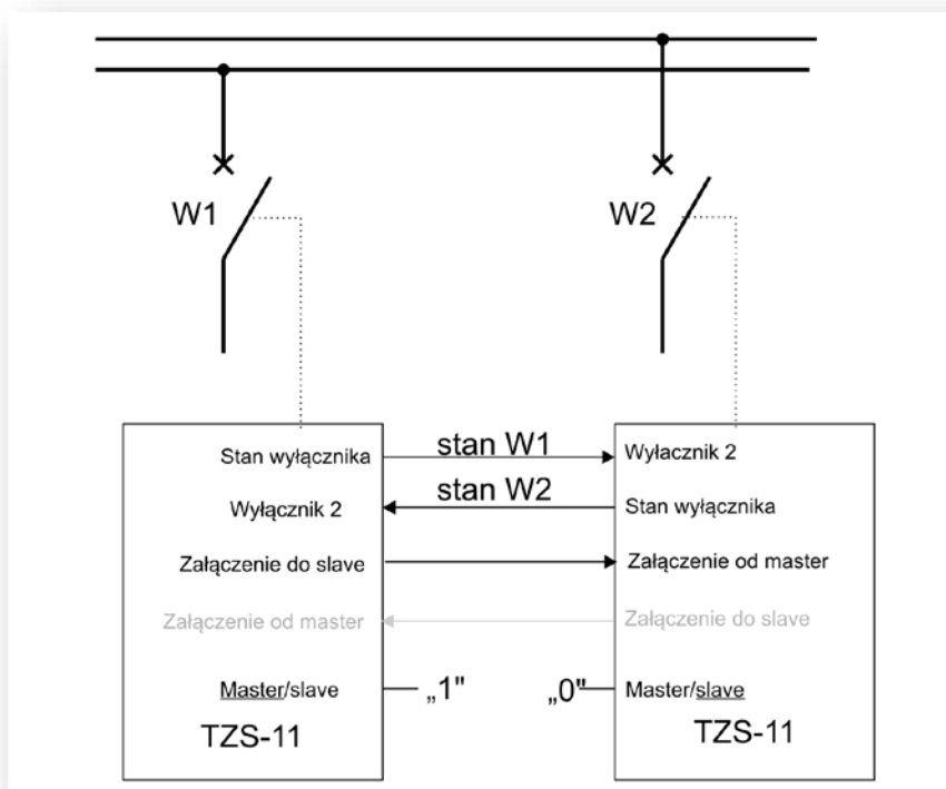
Rys. 7.2. Podłączenie urządzeń w trybie master/ slave.
