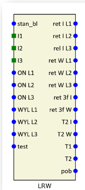
Rys. 7.21. Blok logiczny funkcji LRW.
