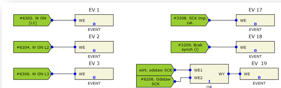
Rys. 7.42. Przykładowa konfiguracja funkcji rejestratora zdarzeń.
