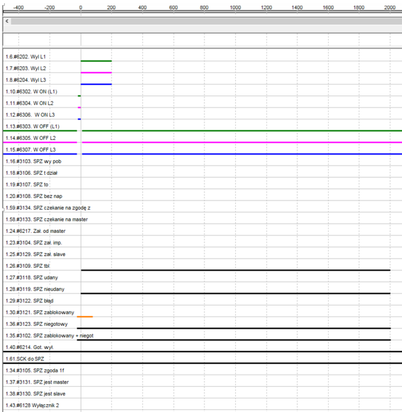
Rys. 7.11. Załączenie przez zwarcie.
