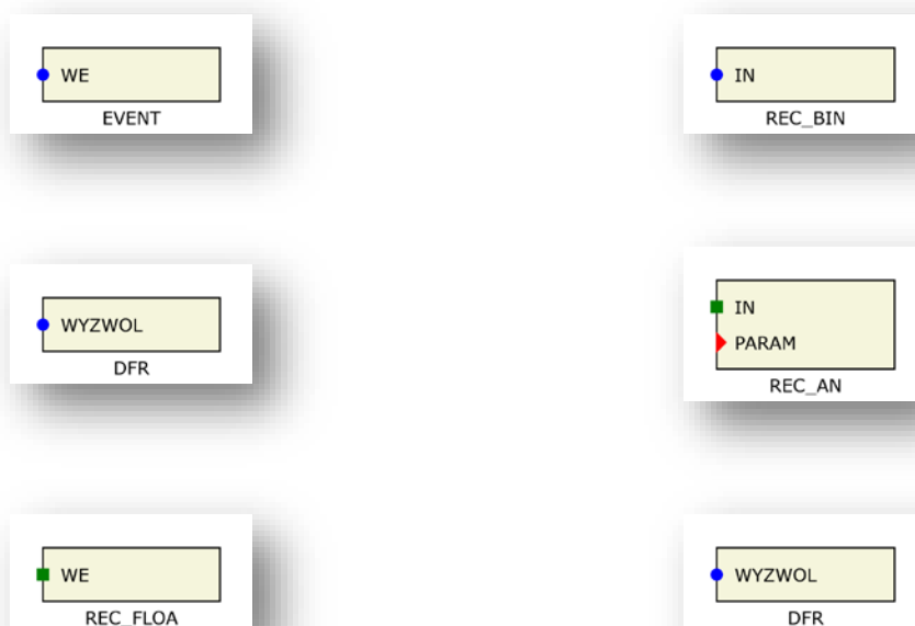
Rys. 9.46. Blok logiczny dla grupy „registratory”.
