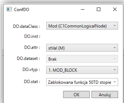
Rys. 7.58. Przypisywanie zdarzeń do atrybutu stVal w danej MOD.
