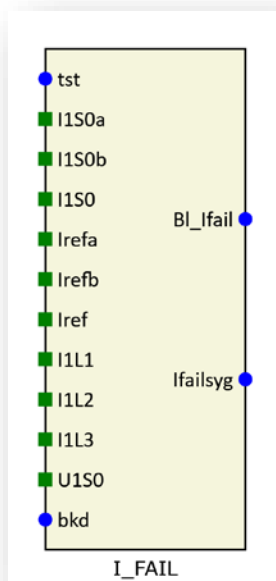
Rys. 7.33. Blok logiczny funkcji I_FAIL.
