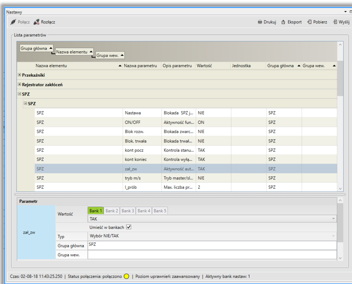
Rys. 9.65. Podgląd nastaw zabezpieczenia – parametr umieszczony w bankach.
