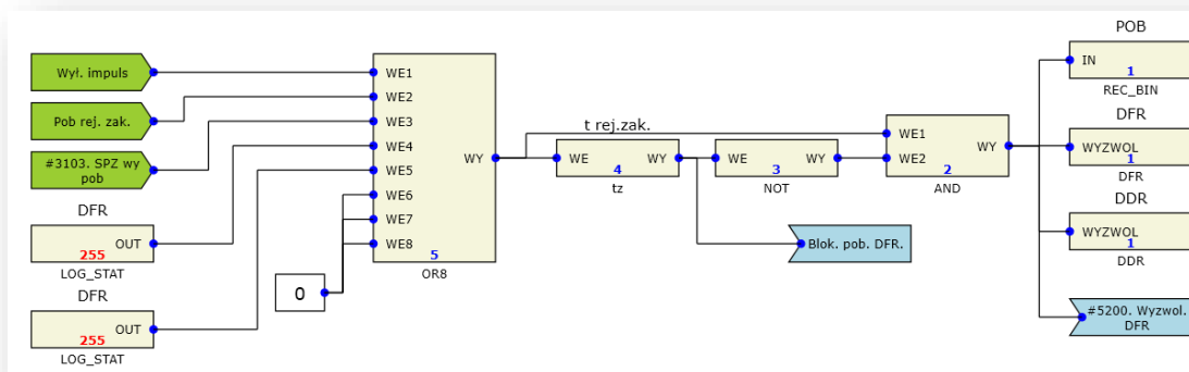
Rys. 7.38. Przykładowa konfiguracja funkcji DFR i DDR.
