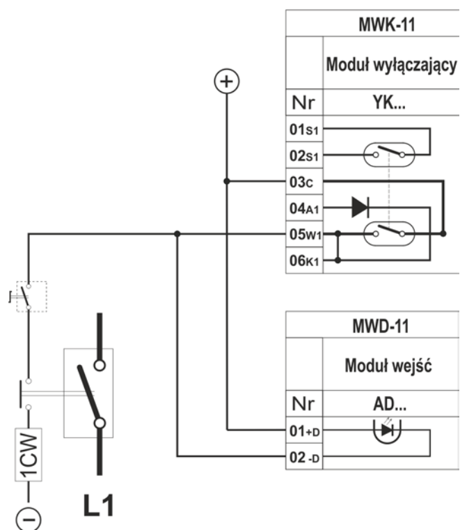
Rys. 7.19. Przykładowe podłączenie wejść w układzie pomiaru drożności obwodów wyłączających.
