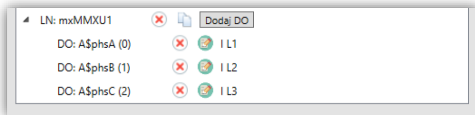
Rys. 7.61. Konfiguracja pomiaru. Wszystkie fazy skonfigurowane.
