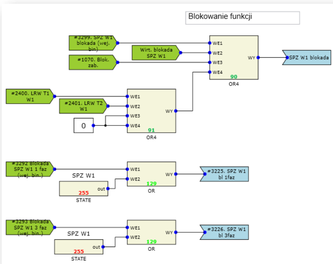
Rys. 7.5. Przykład realizacji blokady funkcji SPZ.
