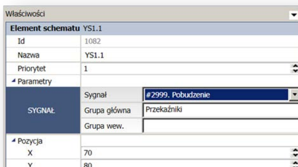
Rys. 9.62. Zmiana sygnału wyjścia binarnego w bloku LOG_STAT.
