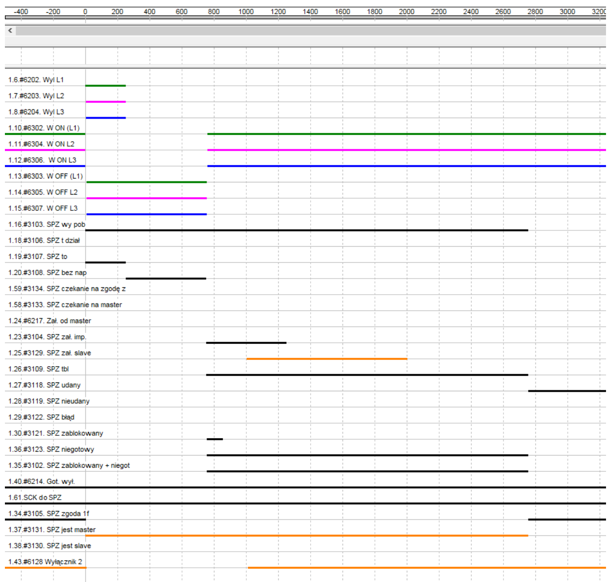
Rys. 7.14. SPZ w układzie z wyłącznikiem prowadzącym (master).
