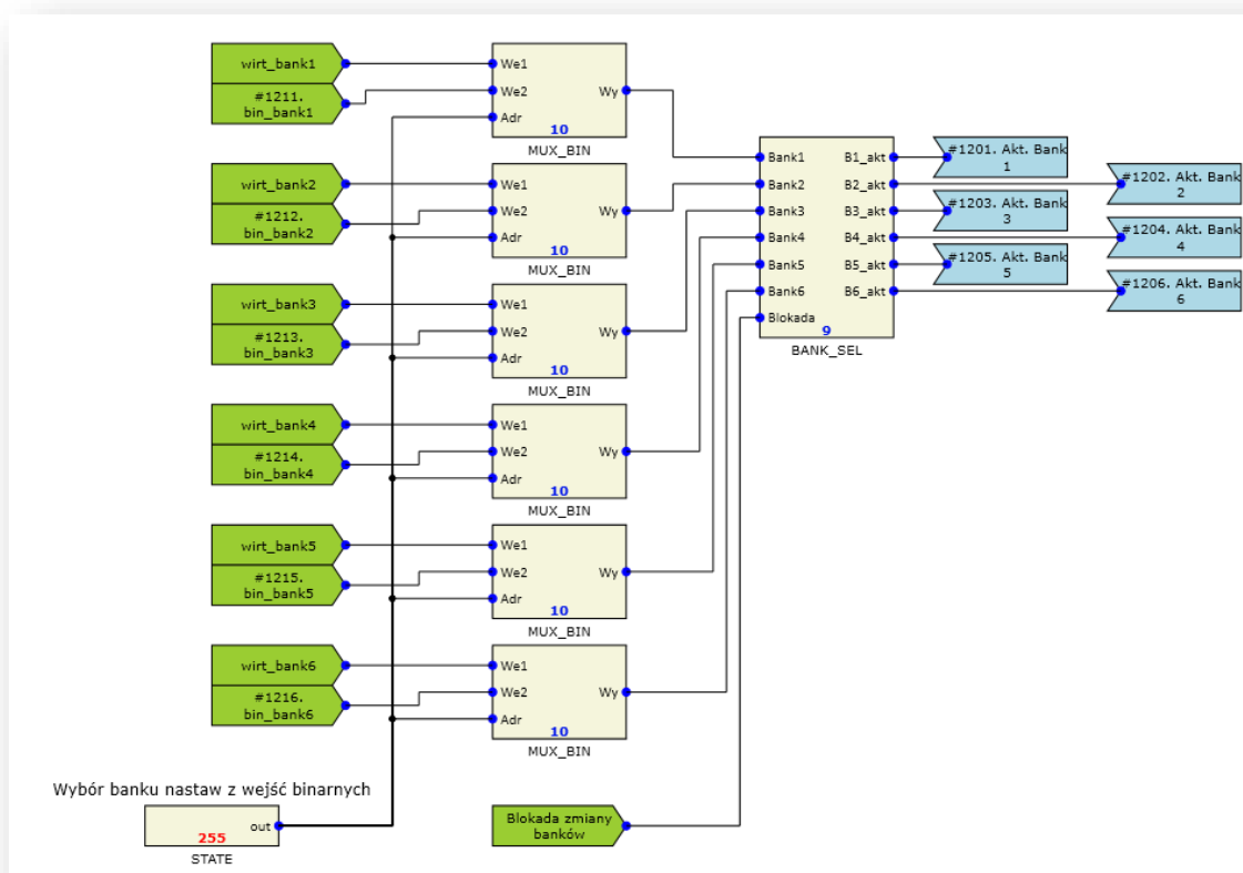
Rys. 7.47. Przykładowa konfiguracja wyboru banku nastaw.
