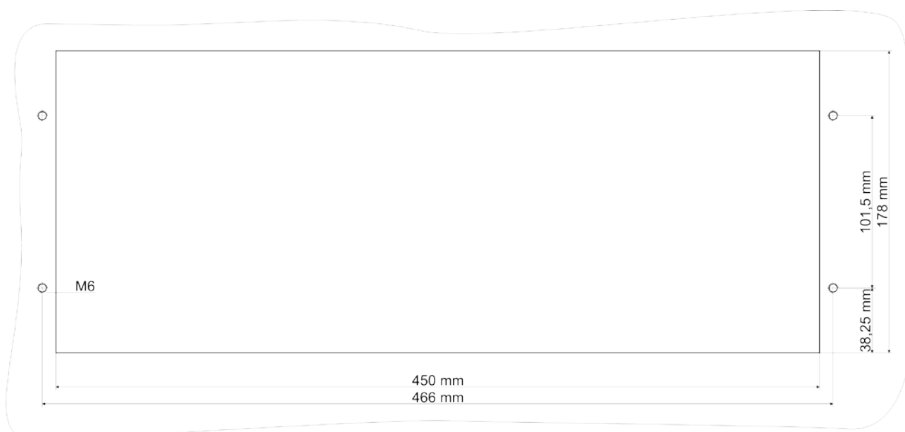
Rys. 11.2. Wytyczne montażowe urządzenia o wysokości 4U.
