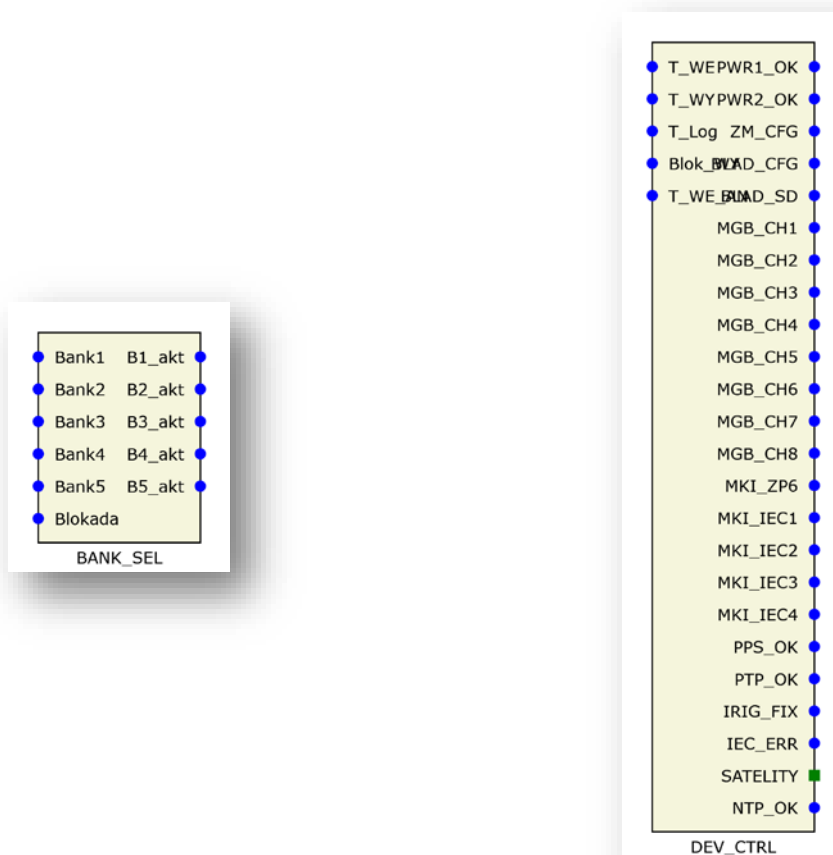
Rys. 9.51. Bloki logiczne dla grupy „f.systemowe”.
