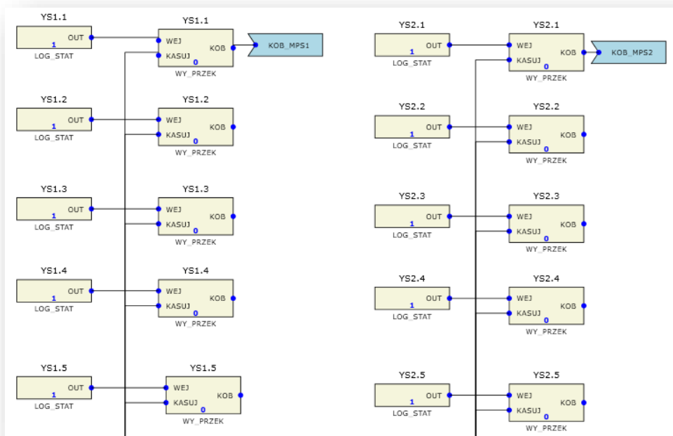
Rys. 9.61. Schemat logiczny, zakładka: „Wyjścia binarne”
