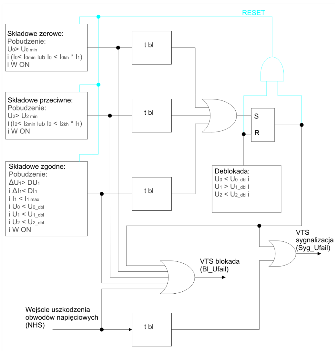
Rys. 7.26 Schemat blokowy działania funkcji VTS.
