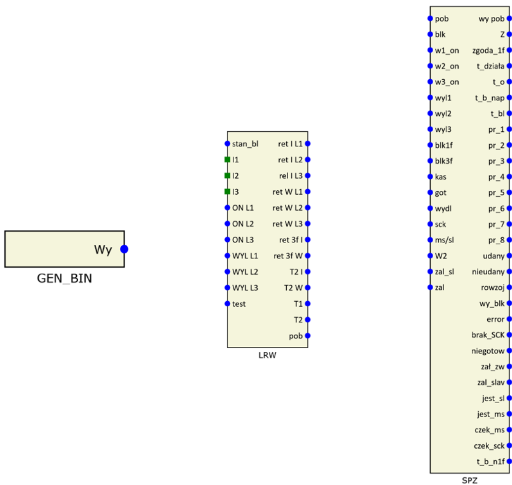
Rys. 9.40. Bloki logiczne dla grupy „automatyka” a) GEN_BIN b) LRW, c) SPZ.
