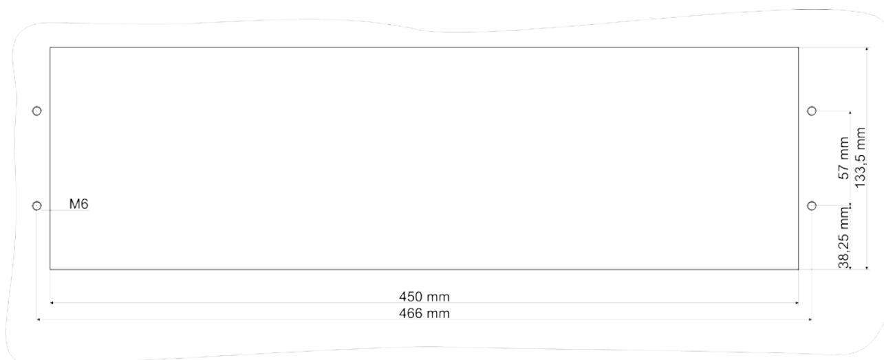
Rys. 11.1. Wytyczne montażowe urządzenia w kasecie Euro 3U.
