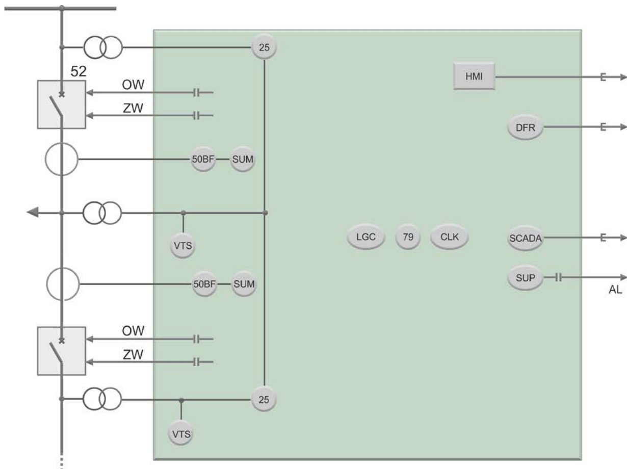
Rys. 3.1. Graficzne przedstawienie funkcji realizowanych przez urządzenie TZS-11.
