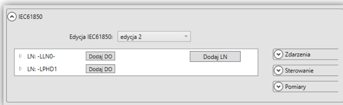
Rys. 7.53. Minimalna konfiguracja IEC61850
