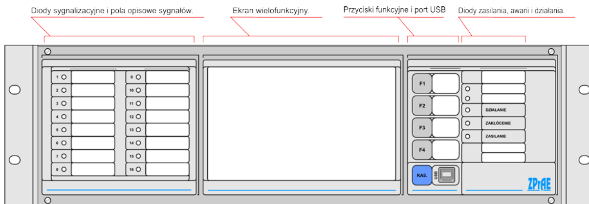
Rys. 4.5. Widok z przodu kasey TZX-11.
