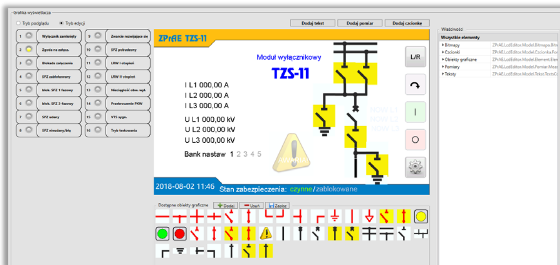
Rys. 9.74. Interfejs graficzny w trybie edycji grafiki wyświetlacza.
