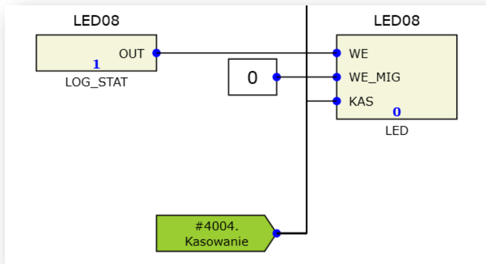
Rys. 7.45. Przykładowa konfiguracja funkcji sygnalizacji lokalnej LED.
