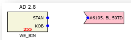
Rys. 9.57. Podłączanie sygnału do wejścia cz.1.
