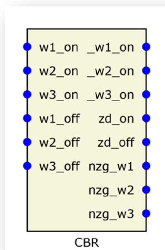
Rys. 7.18. Blok logiczny funkcji CBR.
