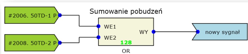
Rys. 9.54. Arkusz schematu logicznego z połączeniami między elementami
