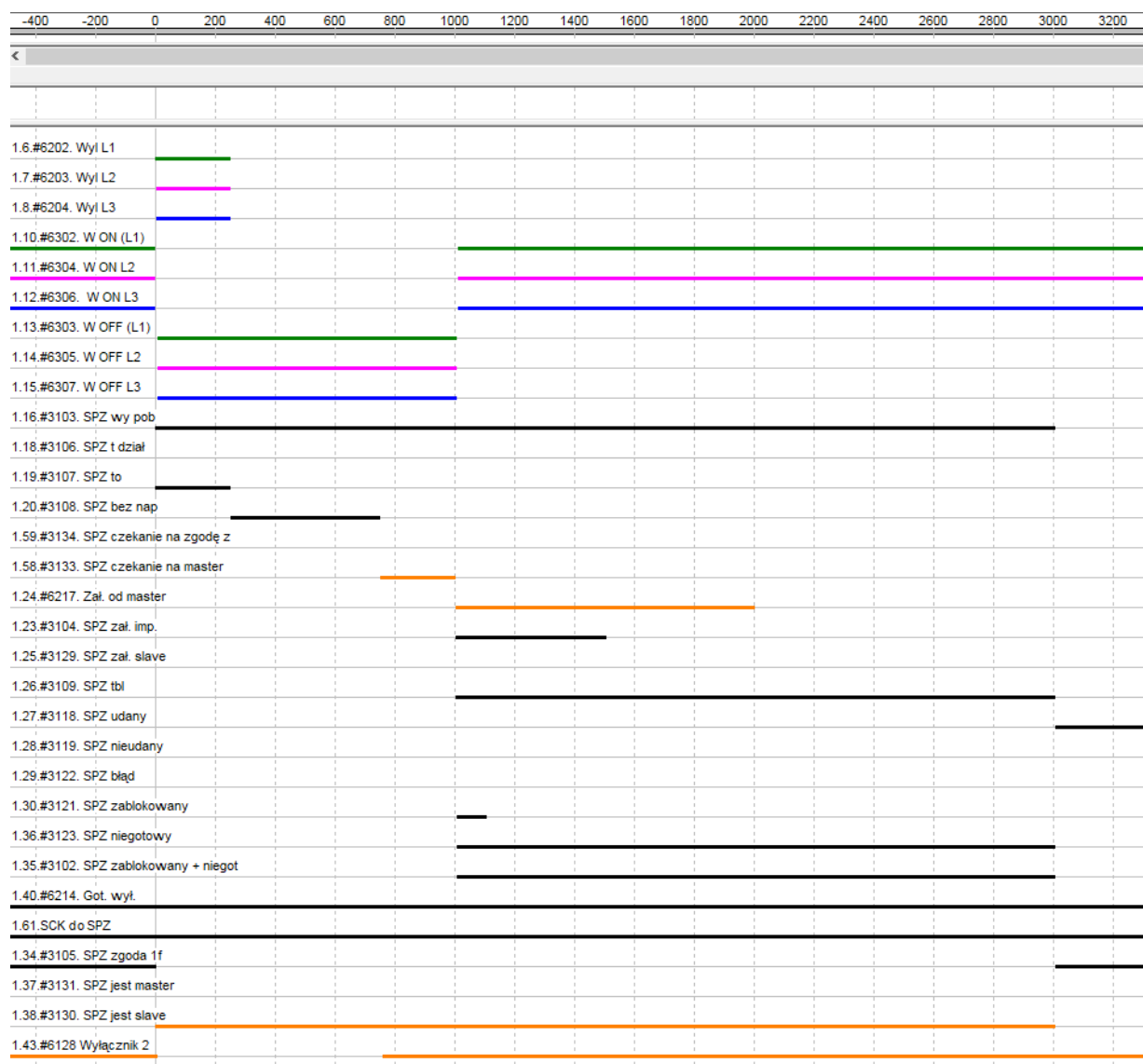
Rys. 7.15. SPZ w układzie z wyłącznikiem podporządkowanym (slave).
