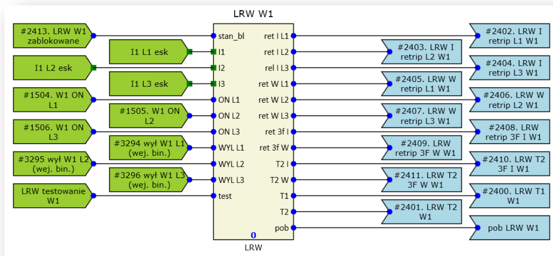
Rys. 7.22. Przykładowa konfiguracja funkcji LRW.
