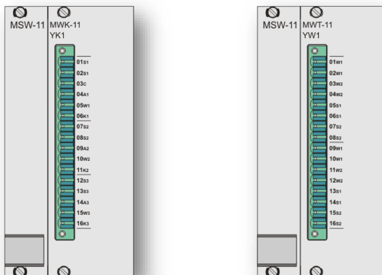
Rys. 5.26. Widok dostępnej dla użytkownika strony modułów wyłączników MFK-11 i trójfazowych MWT-11 wraz z modułem sterującym MSW-11.
