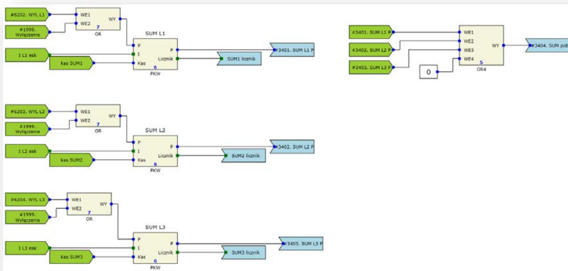
Rys. 7.25. Przykładowa konfiguracja funkcji SUM.
