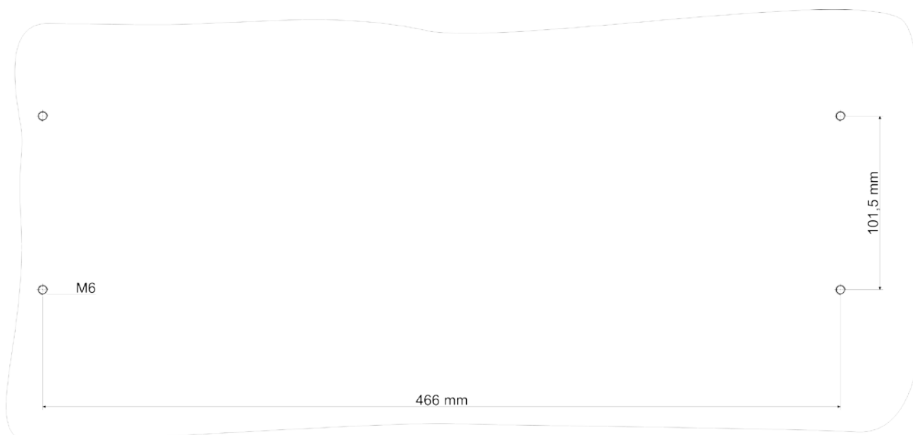
Rys. 11.3. Wytyczne montażowe urządzenia natablicowego o wysokości 4U.
