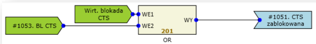
Rys. 7.35. Przykład realizacji blokady funkcji CTS.
