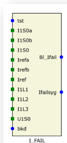
Rys. 9.49. Bloki logiczne dla grupy „f.zabezpiezeniowe” cz. 1.
