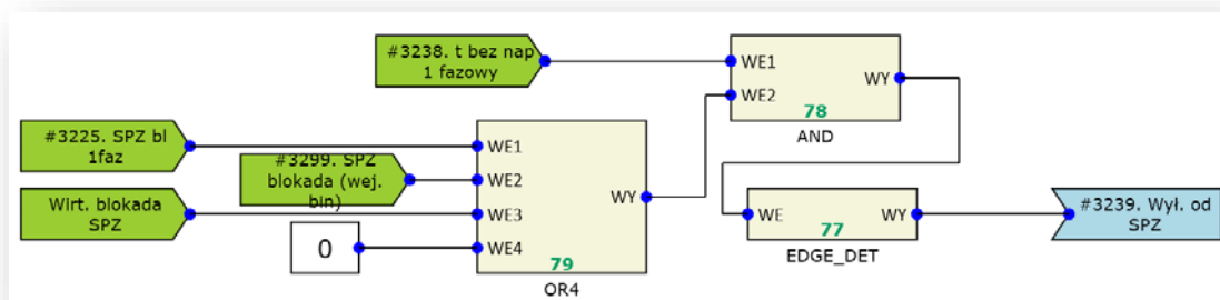
Rys. 7.6. Przykład realizacji automatyki wyłączenia od SPZ po otrzymaniu blokady w czasie przerwy beznapięciowej jednofazowej.
