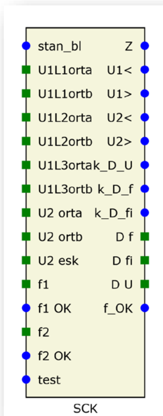
Rys. 7.16. Blok logiczny funkcji SCK.
