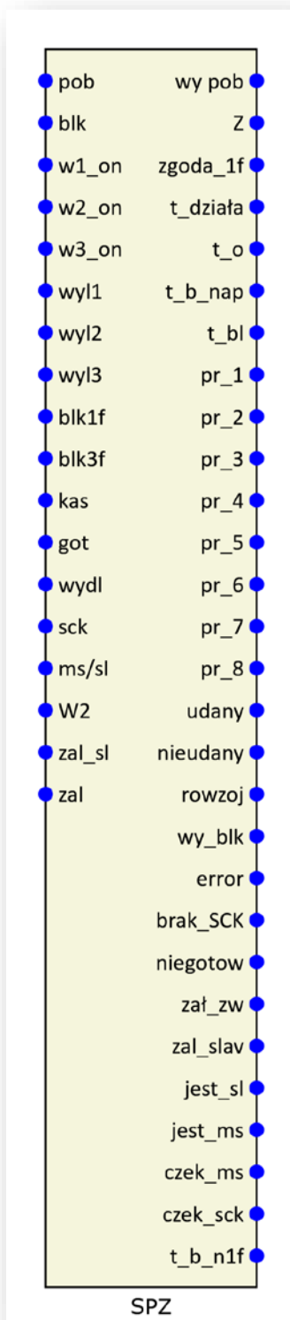
Rys. 7.3. Blok logiczny funkcji SPZ (79).
