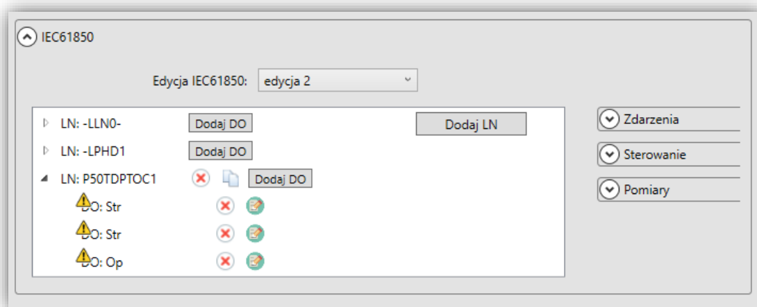
Rys. 7.55. Dodawanie obiektów do węzłów logicznych.
