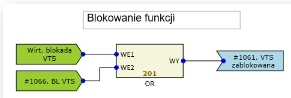
Rys. 7.31. Przykład realizacji blokady funkcji VTS.
