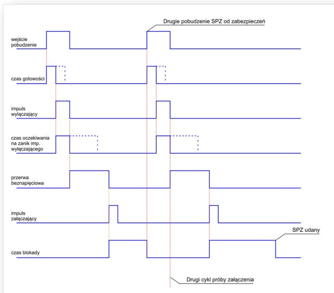
Rys. 7.1. Przebiegi ilustrujące działanie funkcji SPZ (79).
