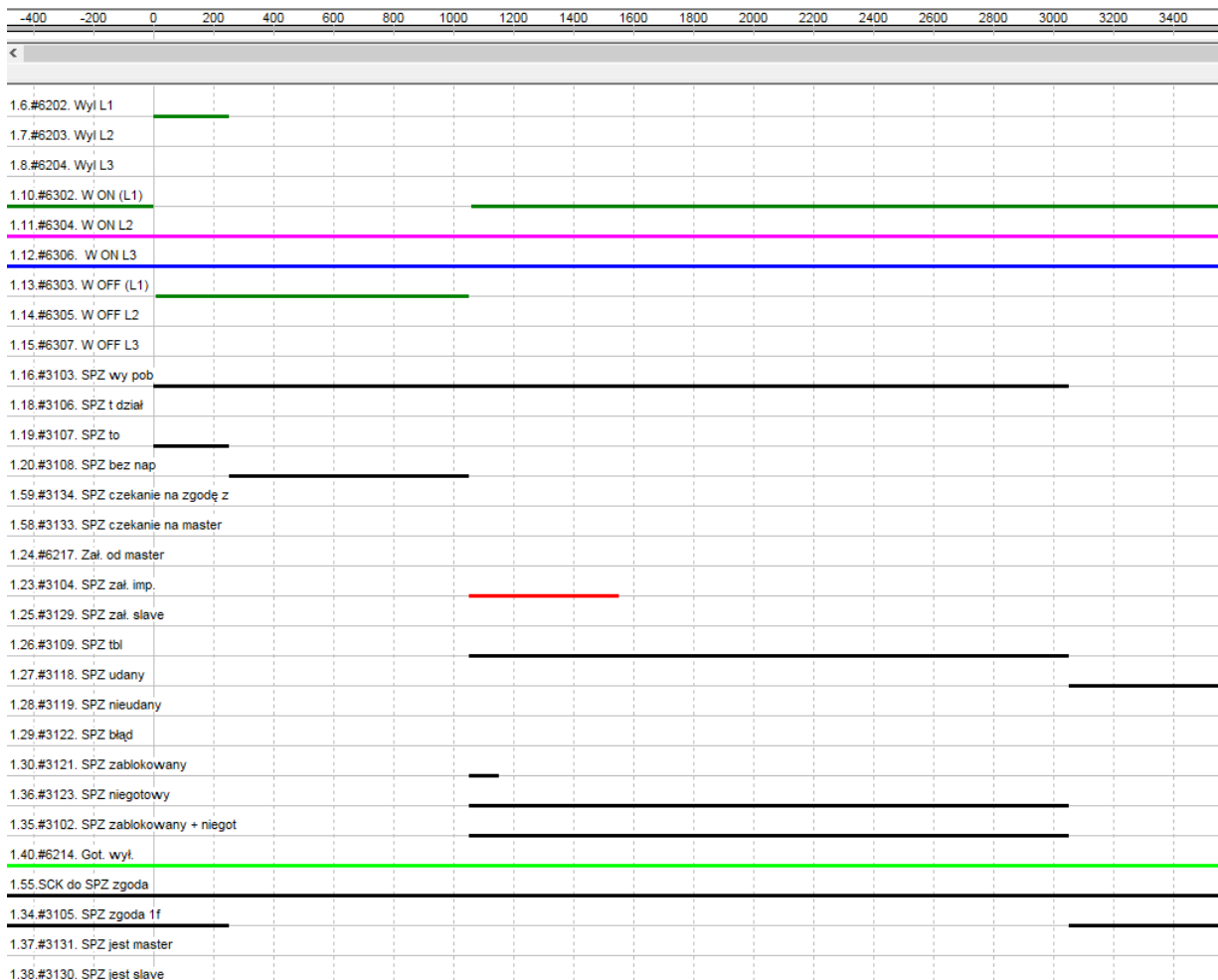
Rys. 7.7. SPZ 1- fazowy
