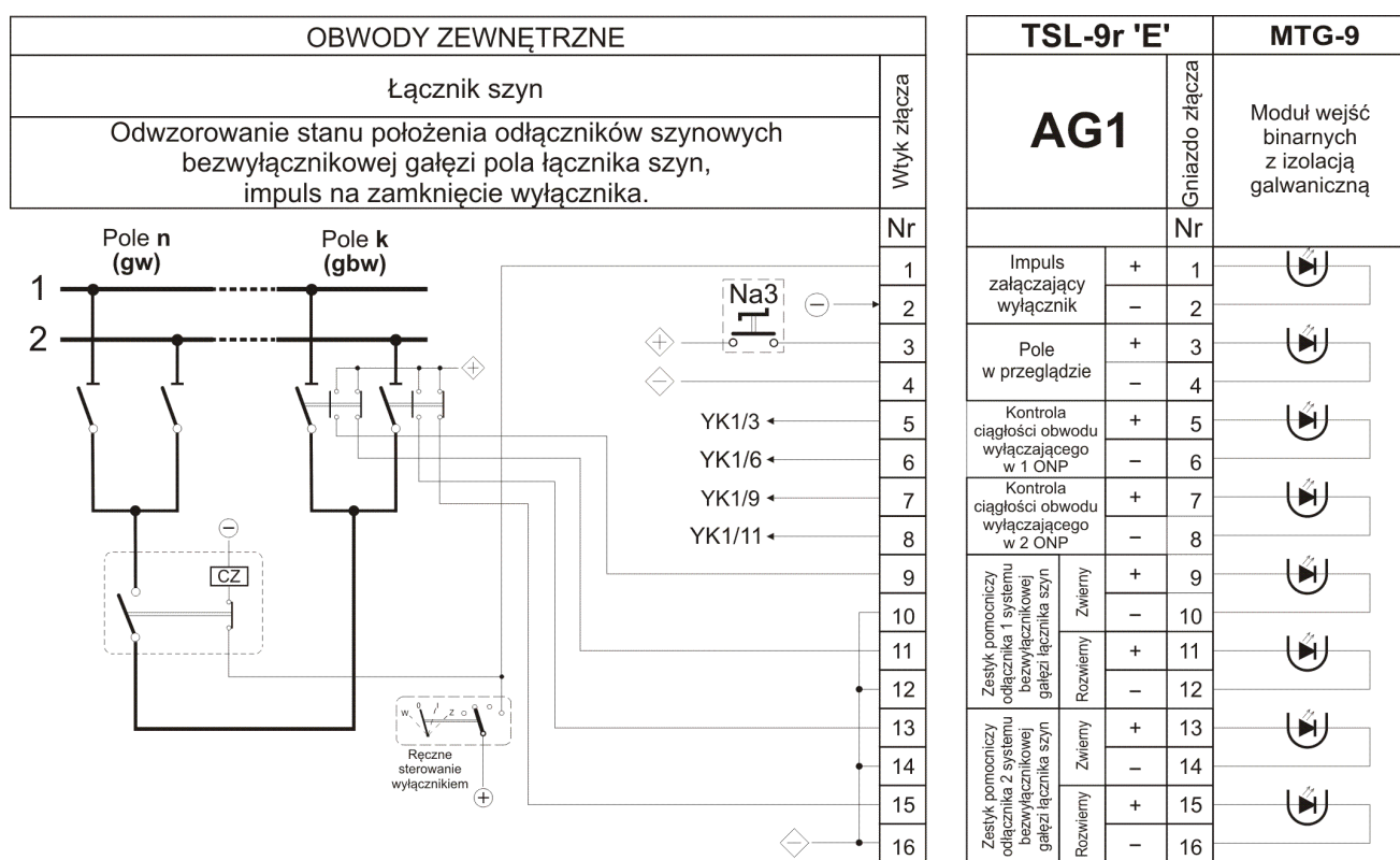
Rys. 10.26. Schemat włączenia obwodów odwzorowania i kontroli ciągłości obwodów wyłączających (2).
