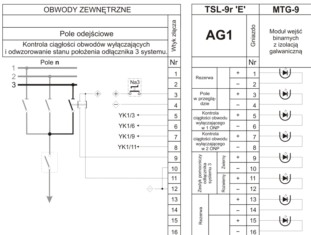
Rys. 10.25. Schemat włączenia obwodów odwzorowania i kontroli ciągłości obwodów wyłączających (1).
