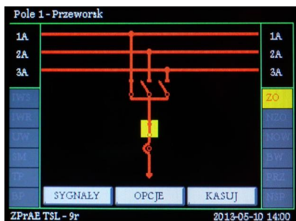
Rys. 4.20. Widok ekranu podstawowego
