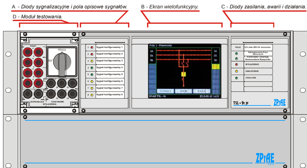
Rys. 4.17. Widok jednostki polowej TSL-9r JP w wersjach B i D.
