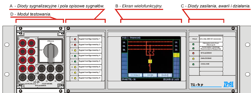
Rys. 4.16. Widok jednostki polowej TSL-9r JP wersjach A, C, AA, AAG.
