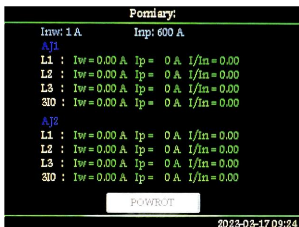
Rys. 4.24. Widok ekranu pomiarów dla jednostki polowej w wersji F
