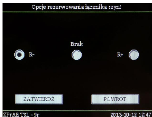
Rys. 11.10. Rezerwowanie pola sposób nr 2 (dla JP w wersji F lub FA) - ustawienia na wyświetlaczu
