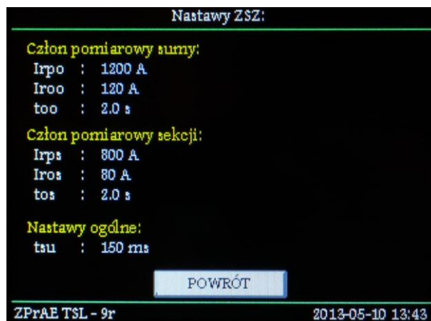
Rys. 4.8. Widok ekranu nastaw ZSZ
