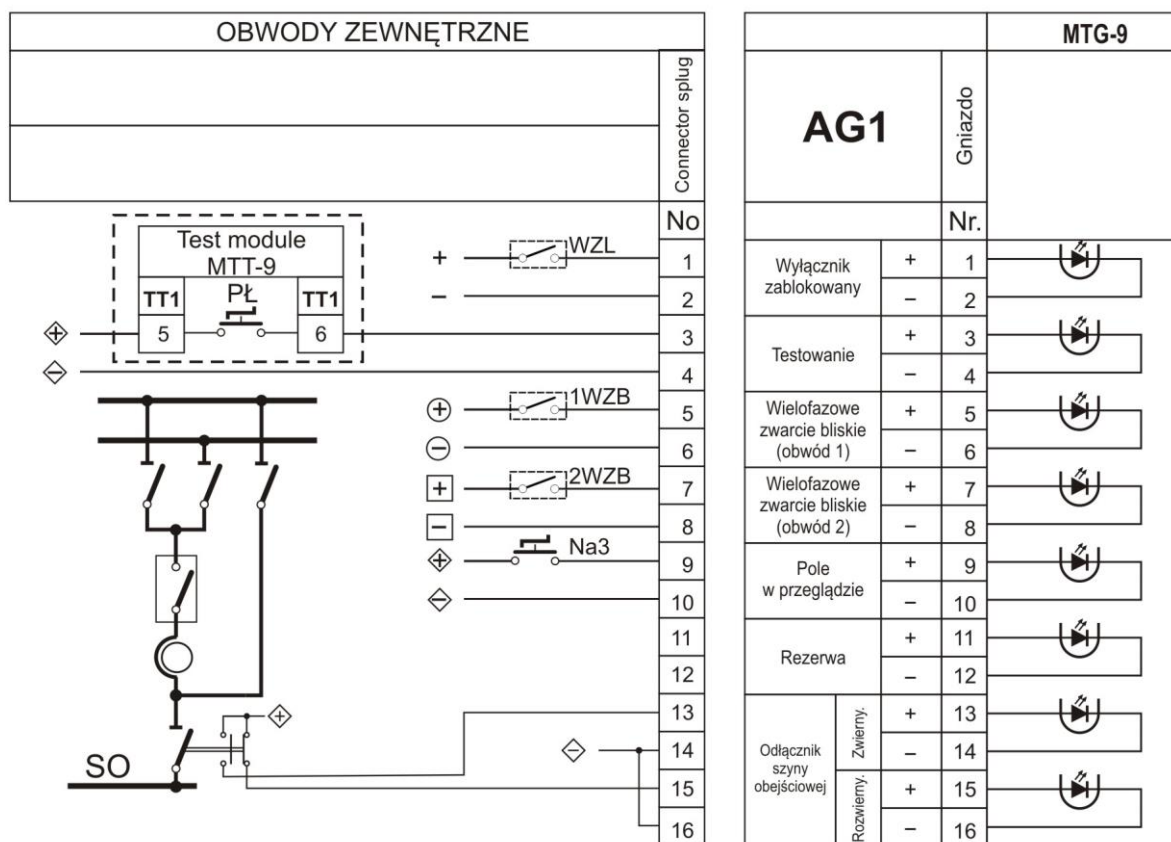
Rys. 10.16. Schemat włączenia obwodów wyłącznik zablokowany, testowania sygnału wielofazowe zwarcie bliskie, pole w przeglądzie i odwzorowania odłącznika szyny obejściowej. (wszystkie wersje poza E i F)
