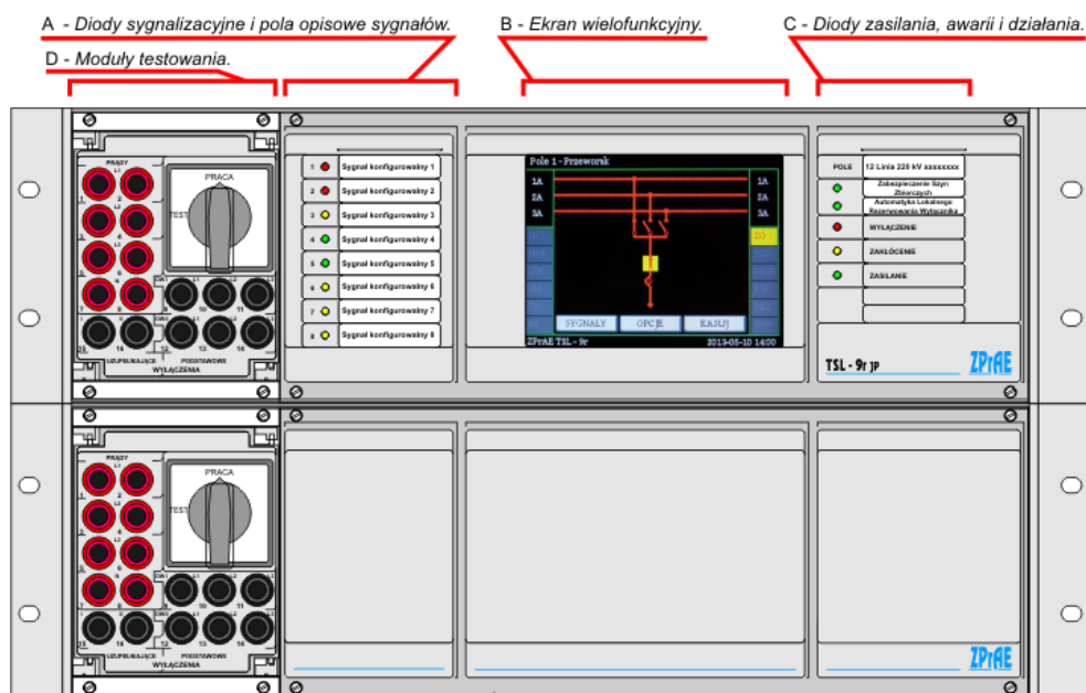
Rys. 4.19. Widok jednostki polowej TSL-9r JP w wersji F.
