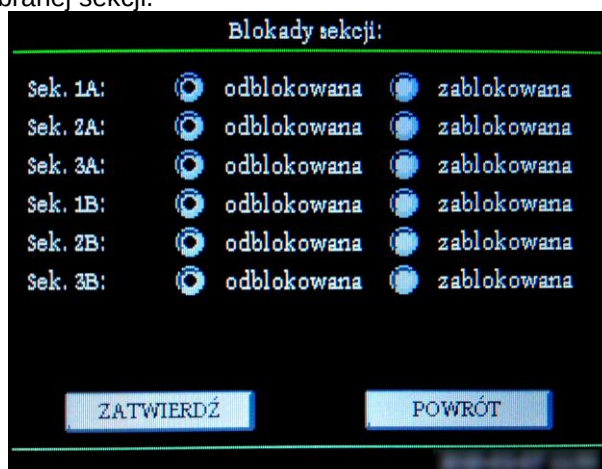
Rys. 11.12. Okno blokad sekcji na wyświetlaczy LCD jednostki centralnej.
