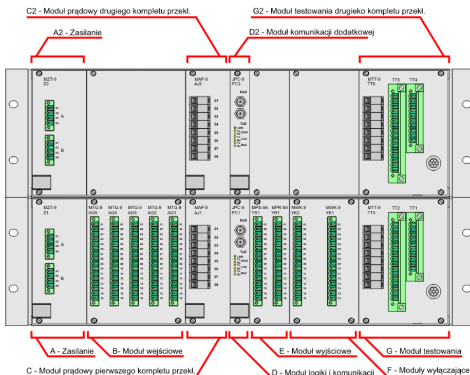
Rys. 4.36. Rozmieszczenie złącz na tylnej płycie jednostki polowej TSL-9r JP w wersji FA.
