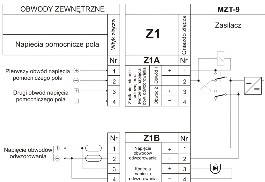
Rys. 10.22. Schemat włączenia obwodów zasilania. (wszystkie wersje poza F)
