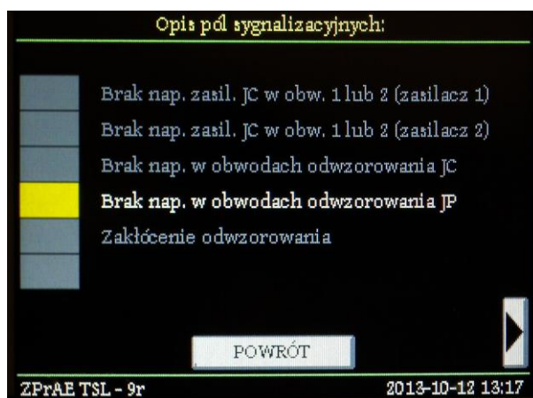
Rys. 4.13. Widok ekranu wybranych sygnałów zakłóceńowych
