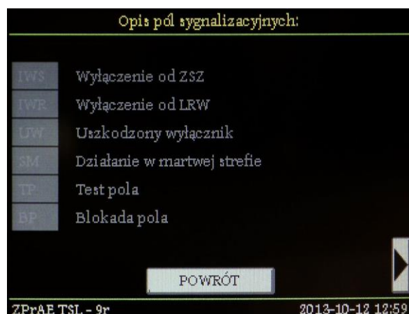
Rys. 4.27. Pierwszy ekran opisu pól sygnalizacyjnych
