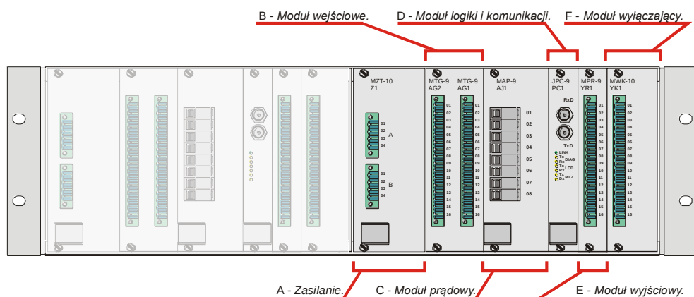
Rys. 4.32. Rozmieszczenie złącz na tylnej jednostki polowej TSL-9r JP w wersji E (dwie w kasecie).
