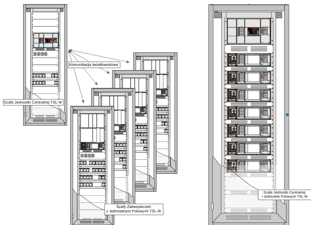
Rys. 4.37. Przykładowe rozmieszczenie jednostek TSL-9r w układzie rozproszonym i scentralizowanym
