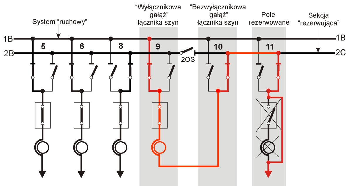
Rys. 11.3. Rezerwowanie pola sposób nr 1
