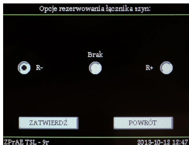
Rys. 11.6. Rezerwowanie pola sposób nr 2- ustawienia na wyświetlaczu
