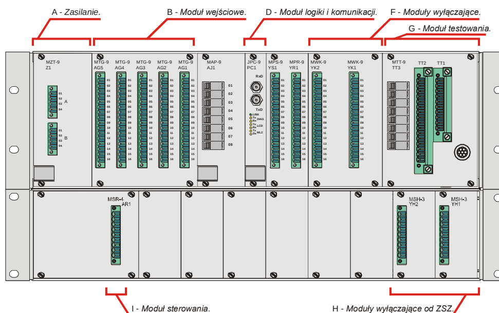
Rys. 4.31. Rozmieszczenie złącz na tylnej płycie jednostki polowej TSL-9r JP w wersji D.
