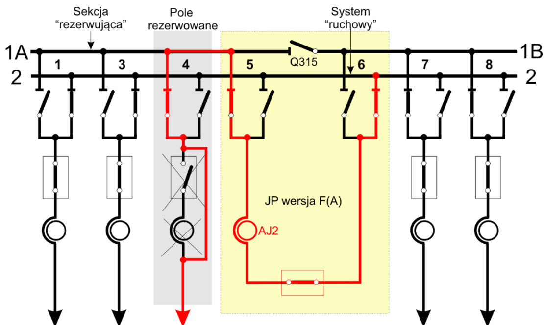
Rys. 11.9. Rezerwowanie pola sposób nr 2 (dla JP w wersji F lub FA)
