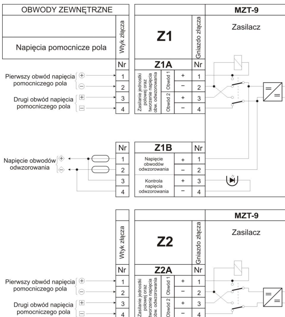
Rys. 10.23. Schemat włączenia obwodów zasilania. (wersje F)
