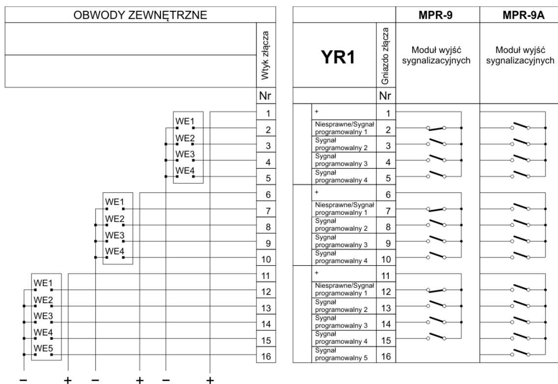
Rys. 10.20. Schematłączenia obwodów sygnalizacji. (wszystkie wersje)
