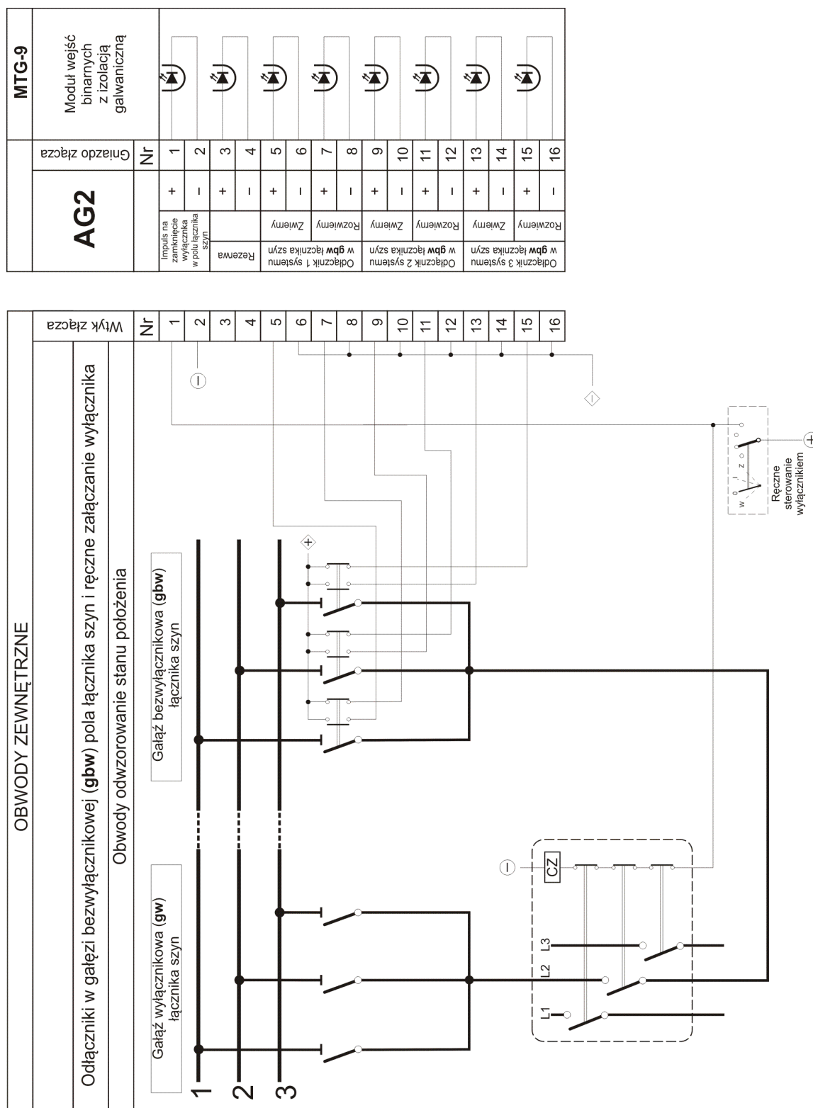
Rys. 10.14. Schemat włączenia obwodów odwzorowania odlącników w gałęzi bezwyłącznikowej i ręczne załączenie wyłącznika. (wszystkie wersje poza E)
