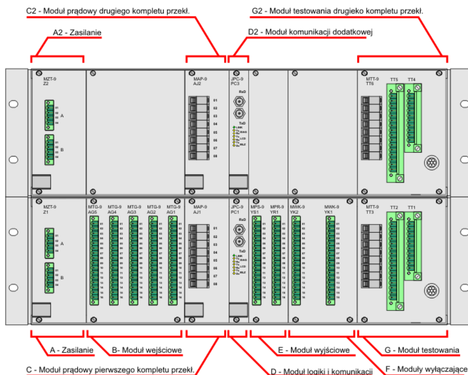
Rys. 4.35. Rozmieszczenie złącz na tylnej płycie jednostki polowej TSL-9r JP w wersji F.
