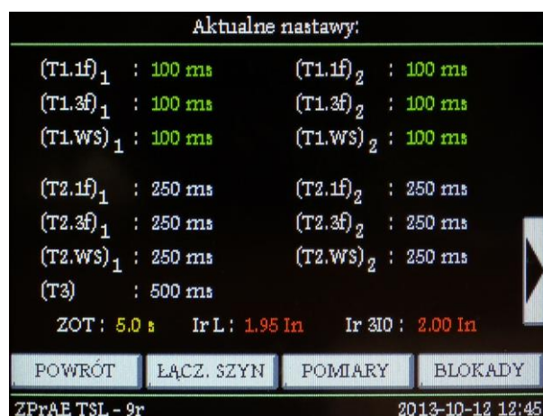
Rys. 4.21. Widok pierwszego ekranu podglądu nastaw
