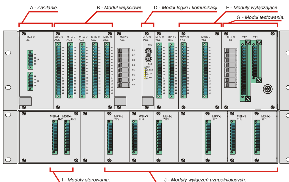
Rys. 4.30. Rozmieszczenie złącz na tylnej płycie jednostki polowej TSL-9r JP w wersji B.
