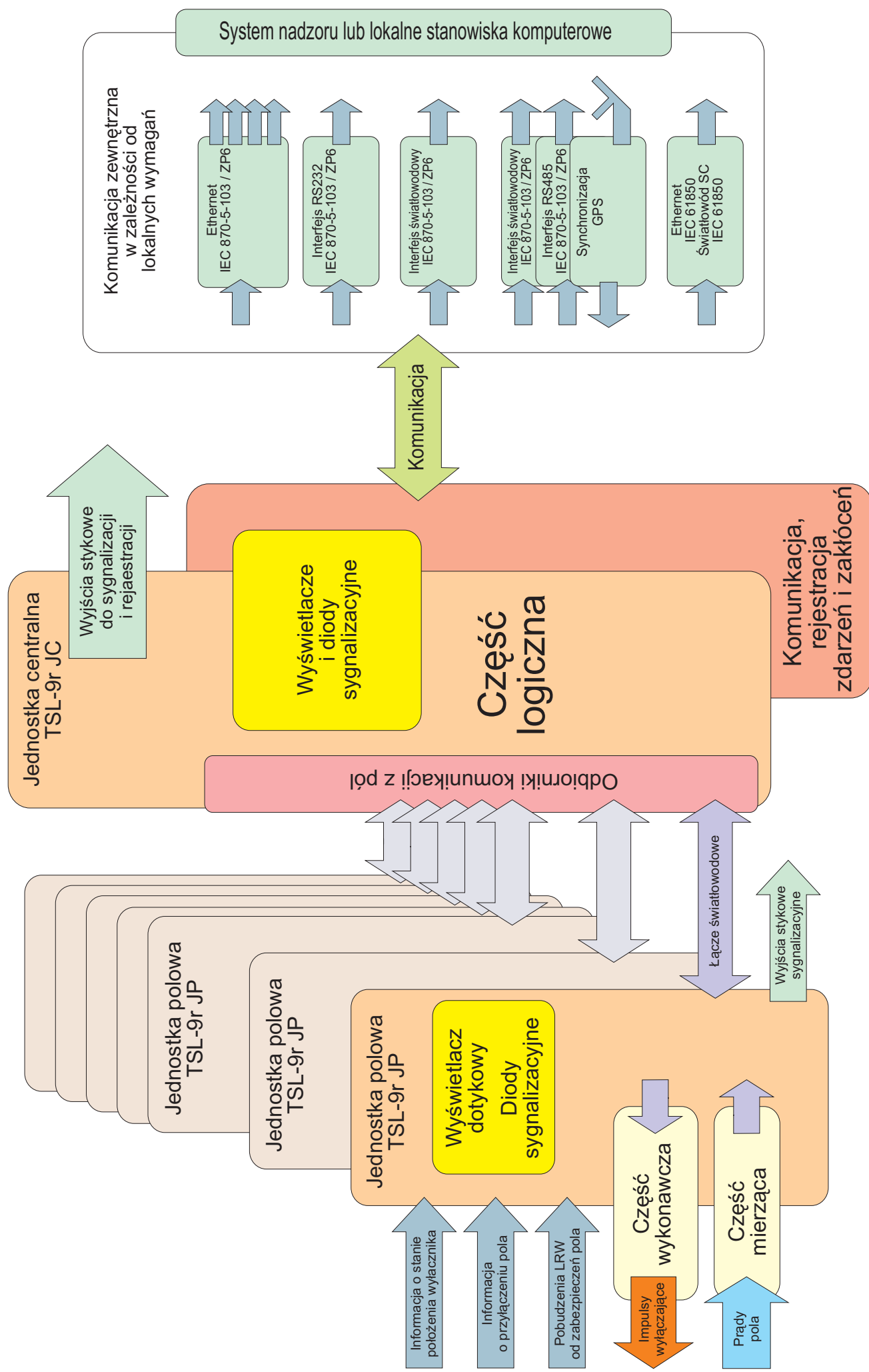
Schemat strukturalny zabezpieczenia ZSZ/LRW typu TSL-9r.
