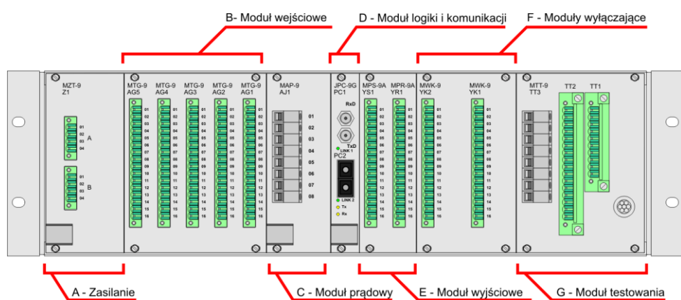
Rys. 4.34. Rozmieszczenie złącz na tylnej płycie jednostki polowej TSL-9r JP w wersji AAG.
