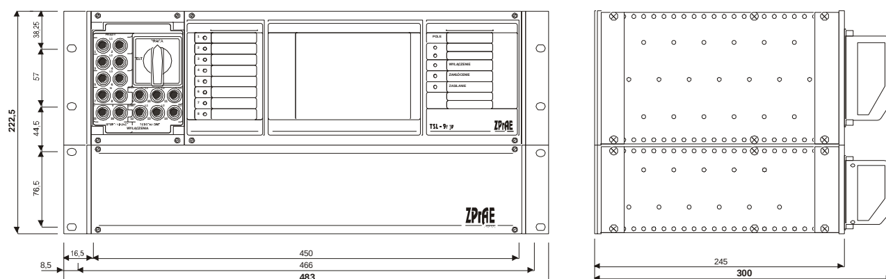
Rys. 4.3. Wymiary zewnętrzne jednostki połowej TSL-9r JP w wersjach B i D.
