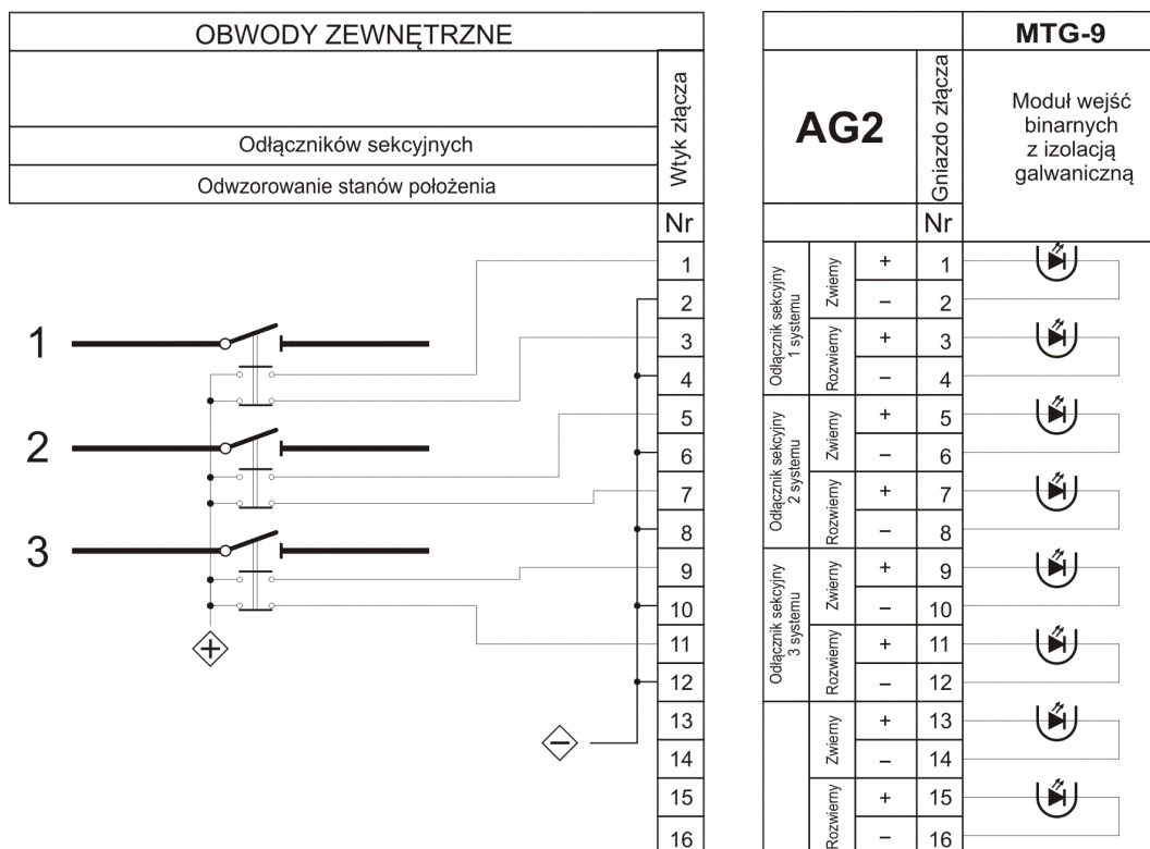
Rys. 10.2. Schemat włączenia obwodów odwzorowania odłączników sekcyjnych
