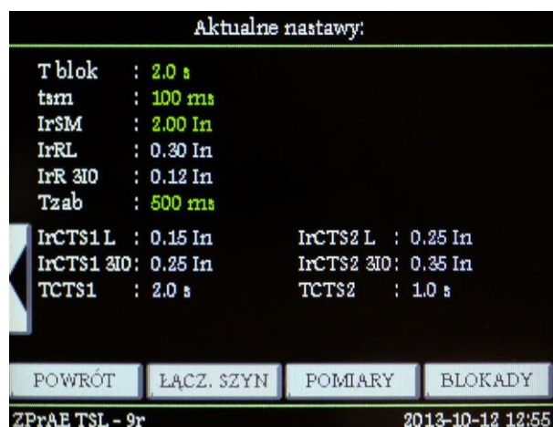
Rys. 4.22. Widok drugiego ekranu podglądu nastaw
