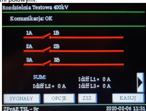
Rys. 4.7. Widok ekranu podstawowego
