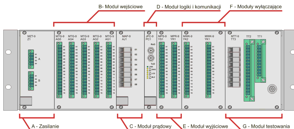
Rys. 4.29. Rozmieszczenie złącz na tylnej płycie jednostki polowej TSL-9r JP w wersji A i C.
