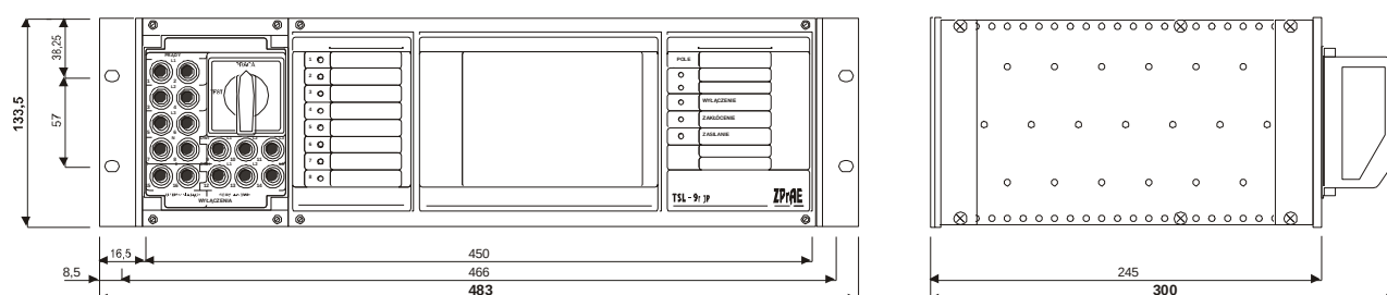
Rys. 4.2. Wymiary zewnętrzne jednostki połowej TSL-9r JP w wersjach A i C.
