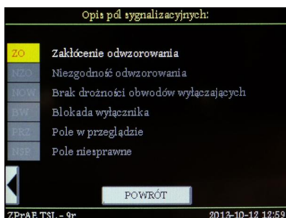
Rys. 4.28. Drugi ekran opisu pól sygnalizacyjnych
