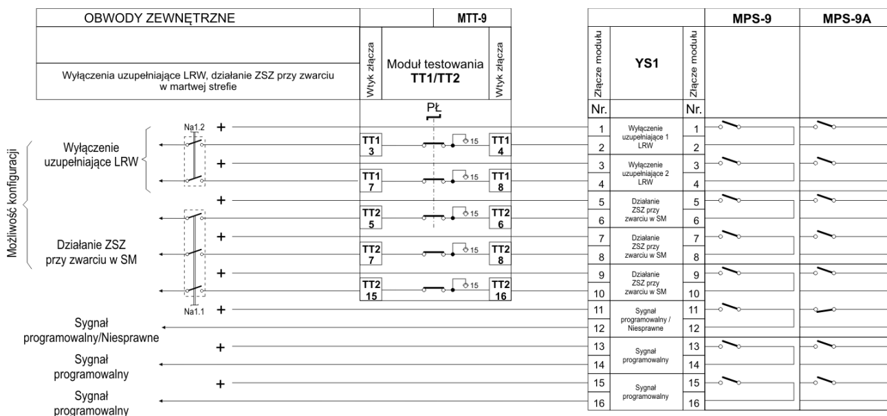
Rys. 10.21. Schematłączenia obwodów włączeń uzupełniających od LRW, działania ZSZ przy zwarcu w martwej strefie i sygnalizacji zaniku napięcia w obwodach odwzorowania. (wszystkie wersje poza E)
