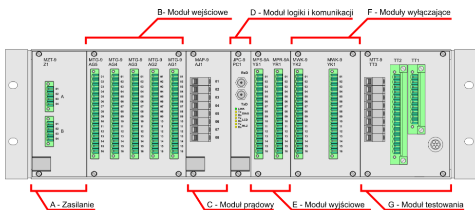
Rys. 4.33. Rozmieszczenie złącz na tylnej płycie jednostki polowej TSL-9r JP w wersji AA.
