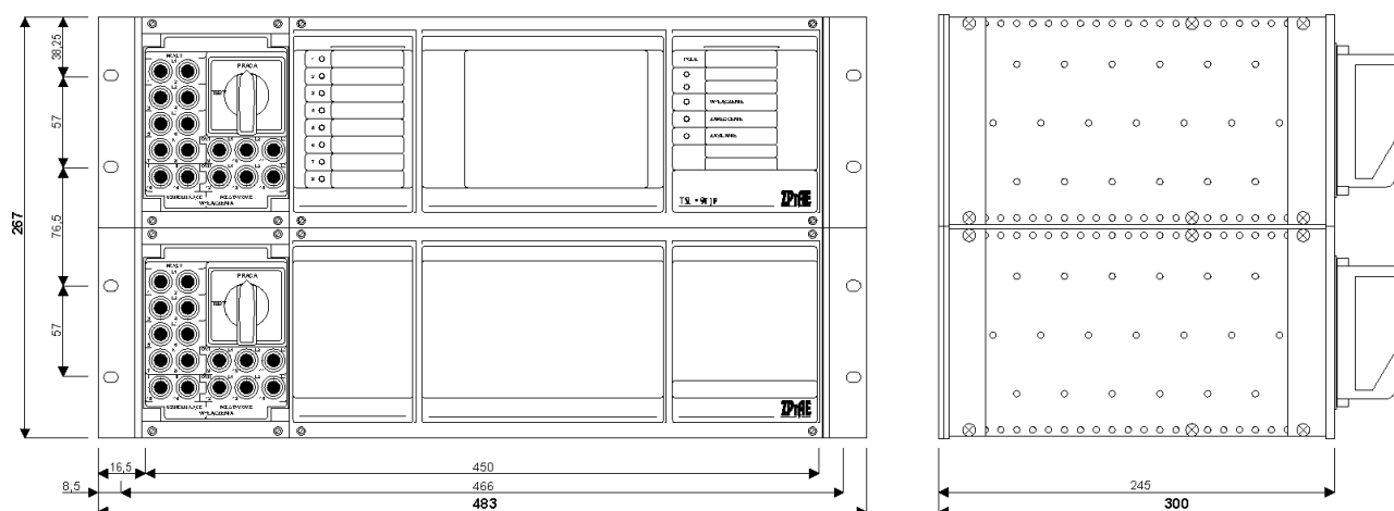
Rys. 4.5. Wymiary zewnętrzne jednostki polowej TSL-9r JP w wersji F.
