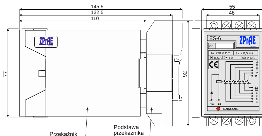
Rys. 2. Rysunek wymiarowy przekaźnika ES-6.
