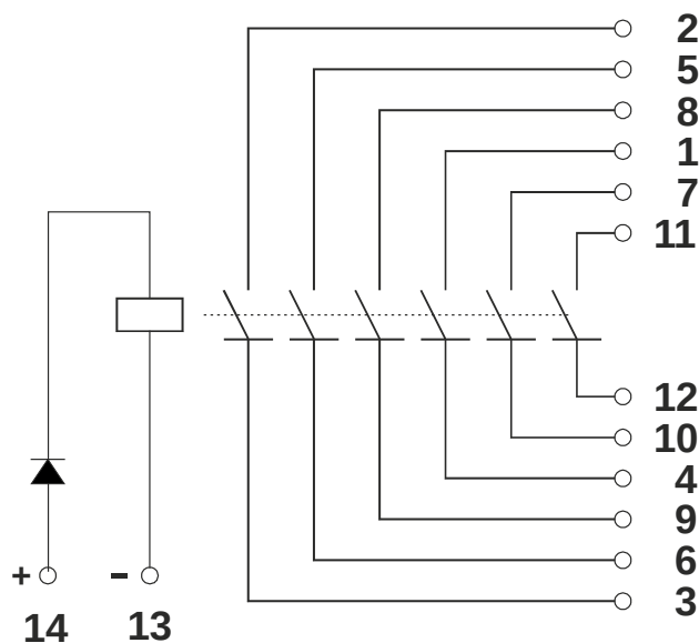
Rys. 1. Przełącznik szybki ES-6 - schemat funkcjonalny wyprowadzeń.
