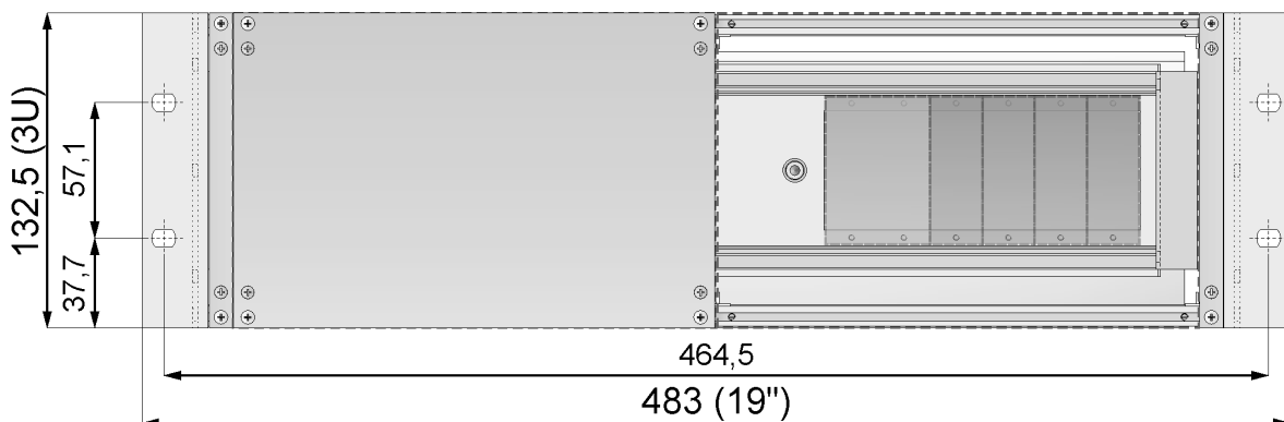
Rys. 1. Wygląd kasety liczników KLQ-2. Widok z przodu.
