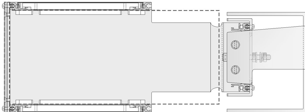
Rys. 3. Wygląd kasety KLQ-2. Widok z boku.
