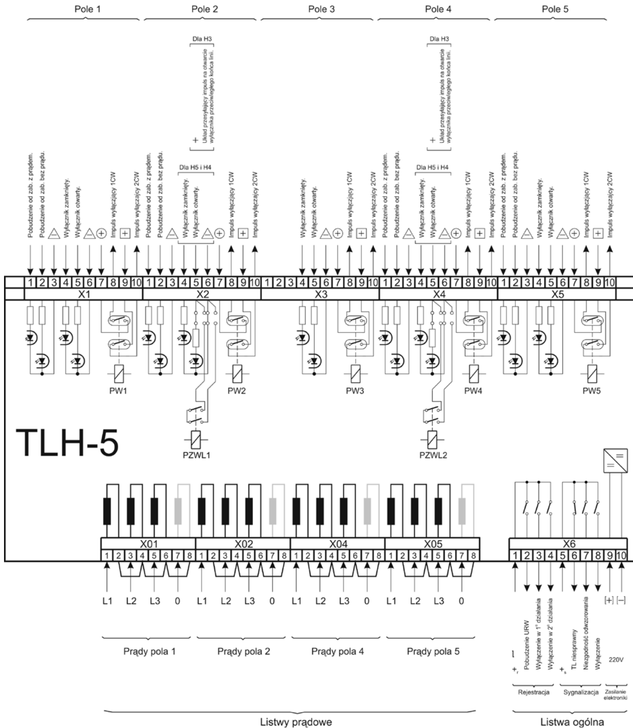
Rys. 8. Schemat funkcjonalny przekaźnika TLH-5.
