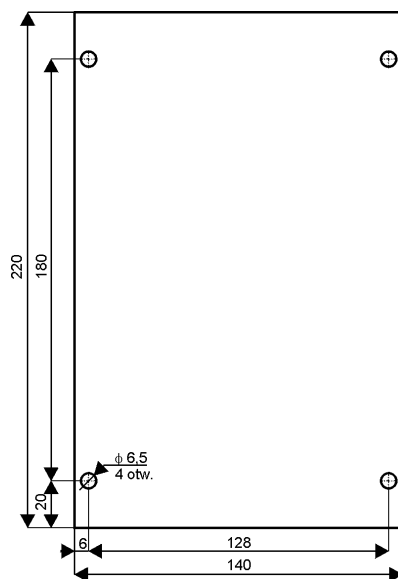
Rys. 4. Zestaw RD-50-30, rozstaw otworów na płycie montażowej.
