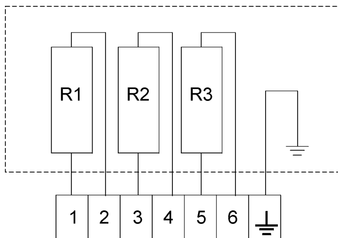
Rys. 2. Listwa zaciskowa zestawu RD-50
