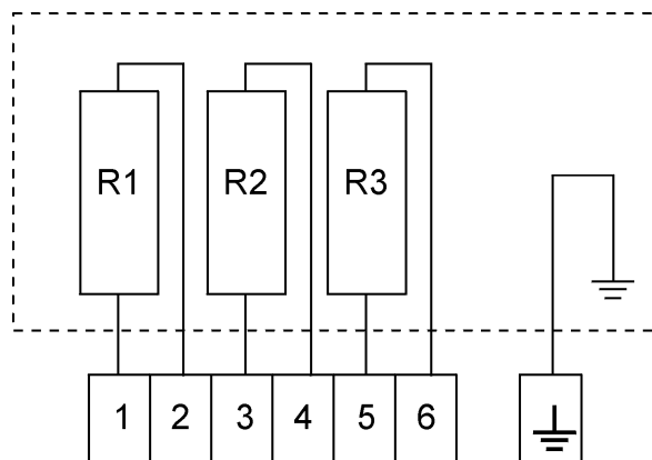
Rys. 5. Listwa zaciskowa zestawu RD-50-30
